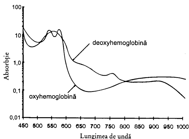
Fig. 12-7. Absorbția luminii (stingere) în funcție de lungimea de undă pentru oxihemoglobină și deoxihemoglobină. (După: Pologe JA: Pulse oximetry: Technical aspects of machine design. Int Anesthesiol Clin 25:137, 1987, cu permisiunea).
