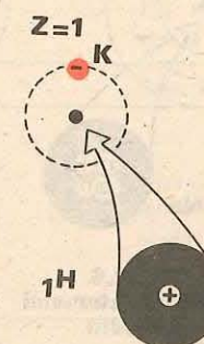
Fig. 2.3. Structura atomului de hidrogen
