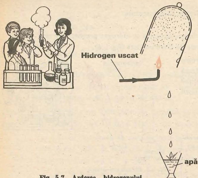
Fig. 5.7. Arderea hidrogenului sub un clopot de sticlă →
