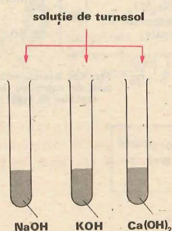
Fig. 8.9. Acțiunea bazelor asupra turnesolului
