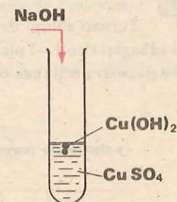
Fig. 8.8. Reacția sulfatului de cupru cu hidroxidul de sodiu
