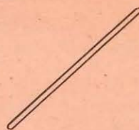
Fig. 1.2.13. Baghetă
