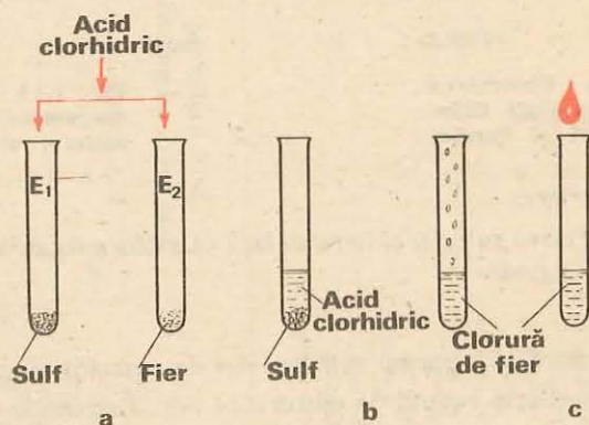
Fig. 1.16. Acțiunea acidului clorhidric asupra sulfurii și fierului
