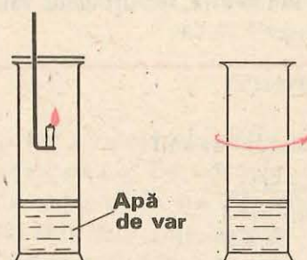
Fig. 8.4. Arderea lumînării în prezența apei de var
