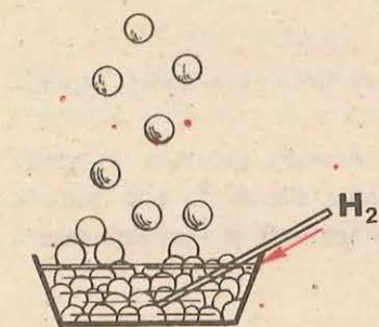
Fig. 5.5. Umplerea baloanelor de săpun cu hidrogen
