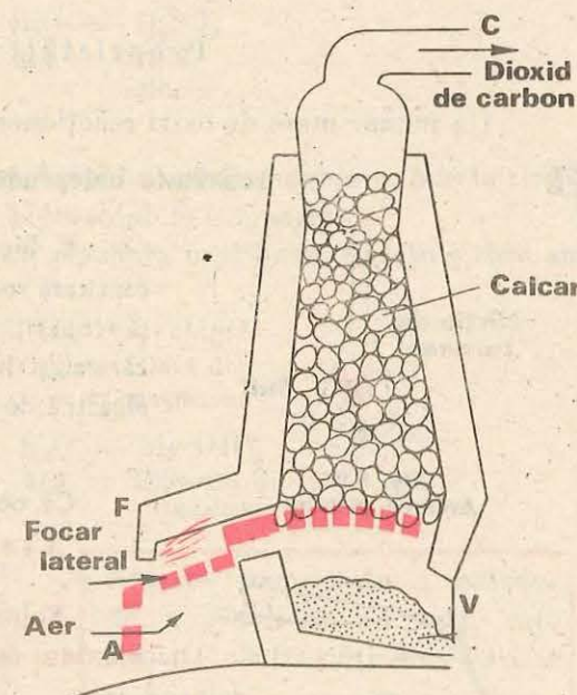
Fig. 8.1. Cuptor de var
