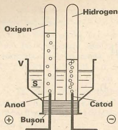
Fig. 4.2. Voltametrul școlar
