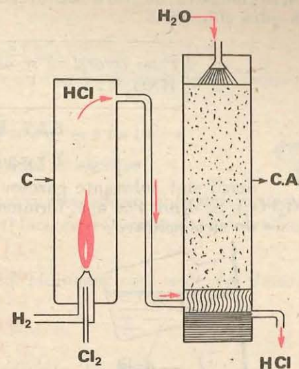
Fig. 8.13. Sinteza industrială a acidului clorhidric
