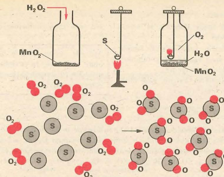
Fig. 4.13. Arderea sulfurului în oxigen
