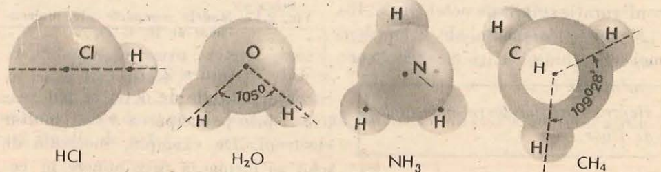
Fig. 2.24 Modele compacte ale moleculelor de \text{HCl} , \text{H}_2\text{O} , \text{NH}_3 și \text{CH}_4
