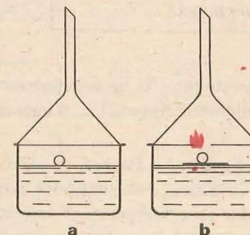
Fig. 5.3. Obținerea hidrogenului prin reacția sodiului cu apa
