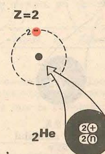
Fig. 2.4. Structura atomului de heliu
