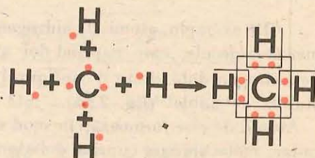
Fig. 2.23. Formarea moleculei de metan
