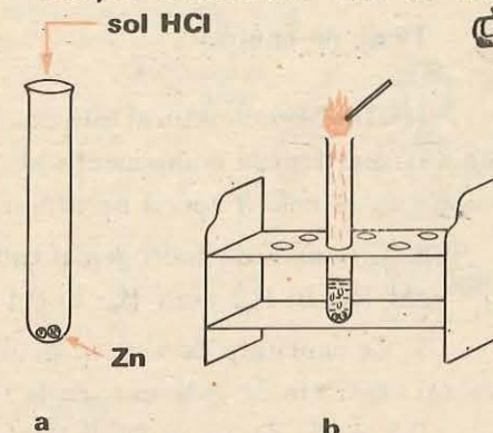
Fig. 5.4. Obținerea hidrogenului prin acțiunea acidului clorhidric asupra zincului
