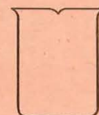
Fig. 1.2.2. Pahare Berzelius
