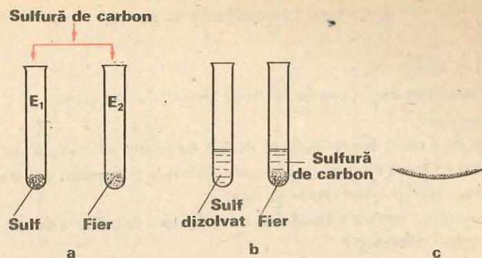
Fig. 1.15. Cercetarea solubilității sulfurii și fierului în sulfură de carbon
