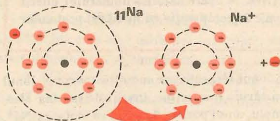
Fig. 2.11. Formarea ionului de sodiu
