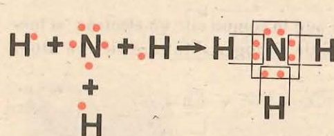
Fig. 2.22. Formarea moleculei de amoniac
