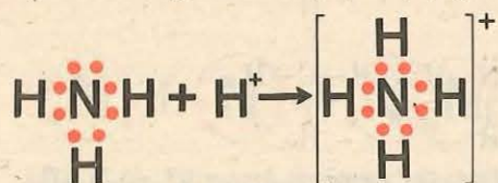
Fig. 2.26. Formarea ionului amoniu
