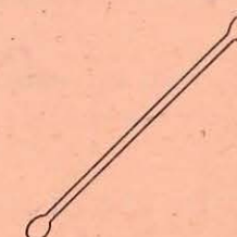
Fig. 1.4.3. Spatulă
