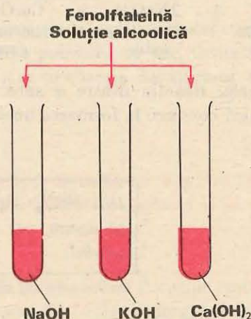
Fig. 8.10. Acțiunea bazelor asupra fenolftaleinei
