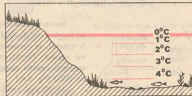
Fig. 6.4. Plătirea gheții pe apă
