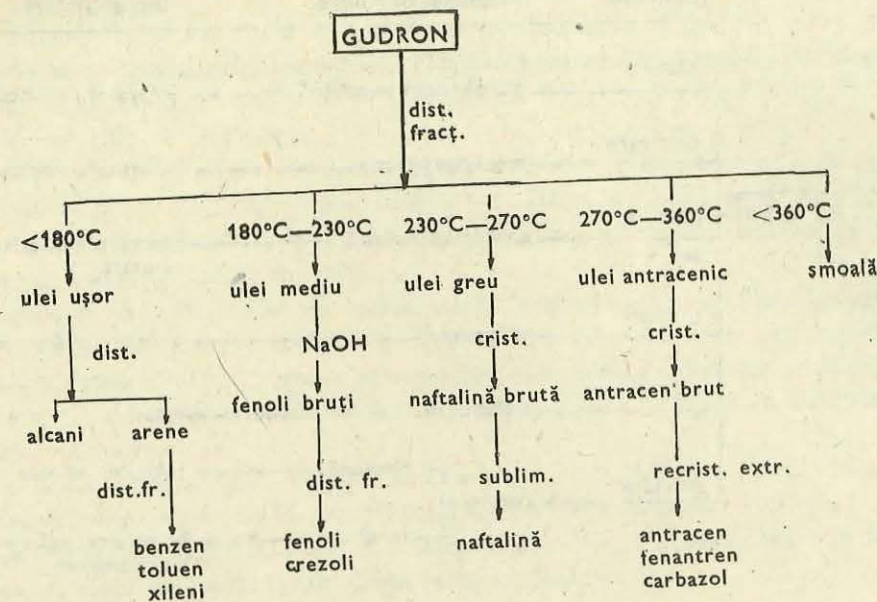
Fig. 27. Schema de prelucrare a gudroanelor de cocserie.
