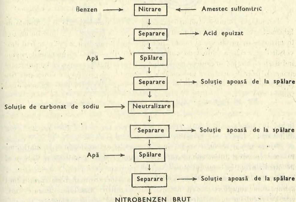
Fig. 15. Schema de operații la fabricarea nitrobenzenului.
