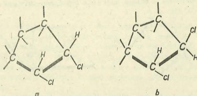
Fig. 8. Schema structurii celor doi izomeri geometrici ai 1,2-diclorciclopentanului: a — izomer cis ; b — izomer trans .
