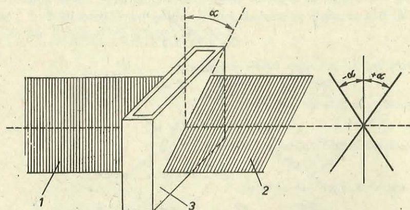
Fig. 9. Rotația luminii polarizate la substanțele optic active:
