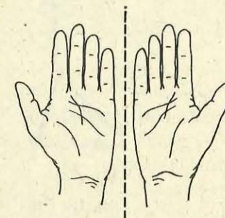
Fig. 10. Cuplu de obiecte enantiomorfe.
