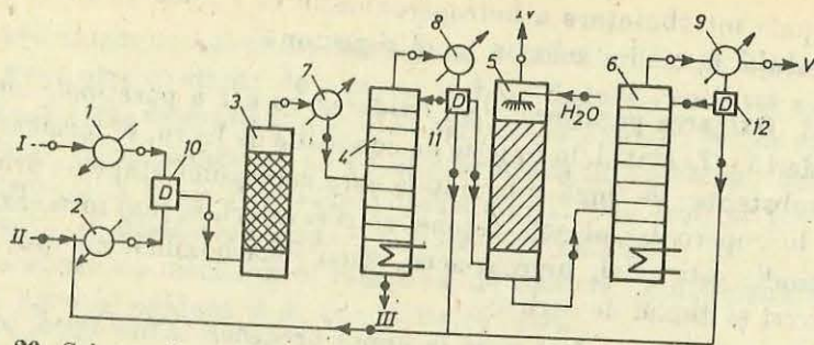
Fig. 20. Schema instalației continue de oxidare a alcoolului metilic. 1, 2 — încălzitor; 3 — reactor de oxidare; 4, 6 — coloane de distilare; 5 — vas de spălare; 7, 8, 9 — condensațoare-răcitoare; 10, 11, 12 — dozatoare; I — aer, II — alcool metilic, III — soluție de aldehydă formică 40%, IV și V — gaze necondensabile.
