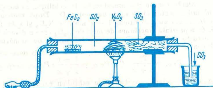
Fig. 4.6. Instalație pentru realizarea reacției de oxidare a SO_2 la SO_3 , pe catalizator de V_2O_5 .
