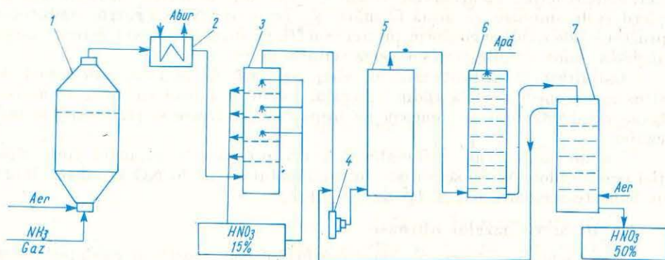
Fig. 4.9. Schema instalației de obținere a acidului azotic.
