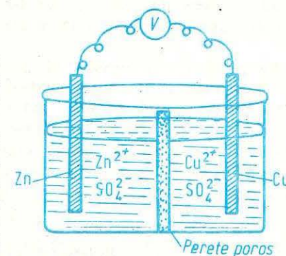
Fig. 1.8. Pila Daniel.
