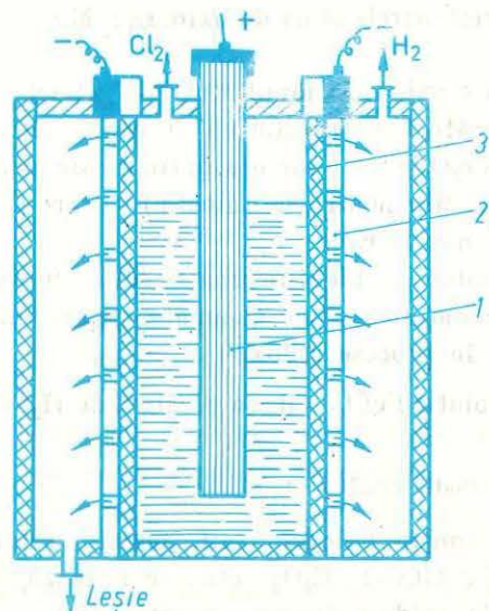
Fig. 1.14. Celula de electroliză cu diafragmă :
