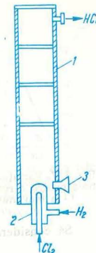
Fig. 3.16. Reactorul pentru obținerea HCl.
