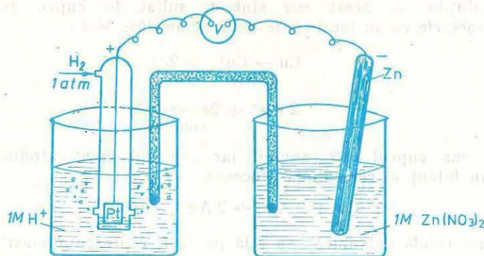
Fig. 1.6. Celulă galvanică construită din electrodul normal de hidrogen și semicelula zincului.
