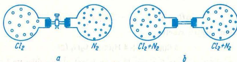
Fig. 2.11. Dispozitiv pentru realizarea unui amestec de două gaze: a — stare inițială (gaze separate); b — stare finală (amestec de gaze).
