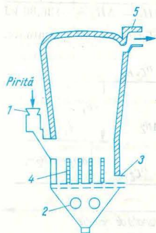
Fig. 2.9. Cuptorul de prăjire a piritei în strat fluidizat.
