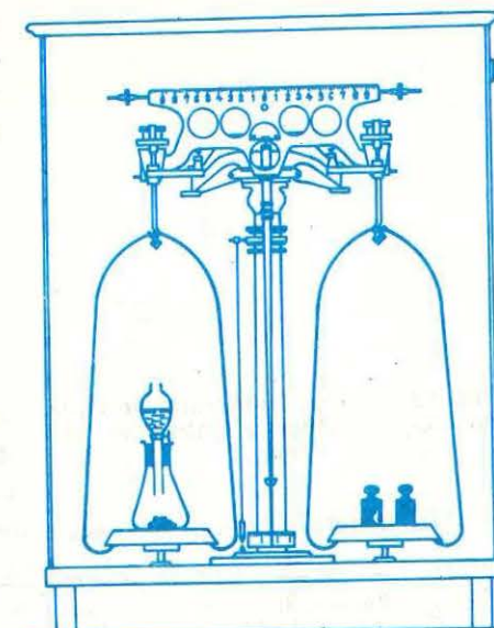
Fig. 3.8. Instalație pentru stabilirea vitezei de reacție.
