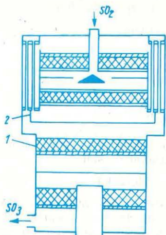
Fig. 4.7. Schema sobei de contact.
