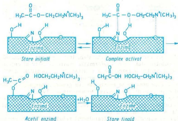
Fig. 3.33. Mecanismul catalizării reacției de hidroliză a acetilcolinei.
