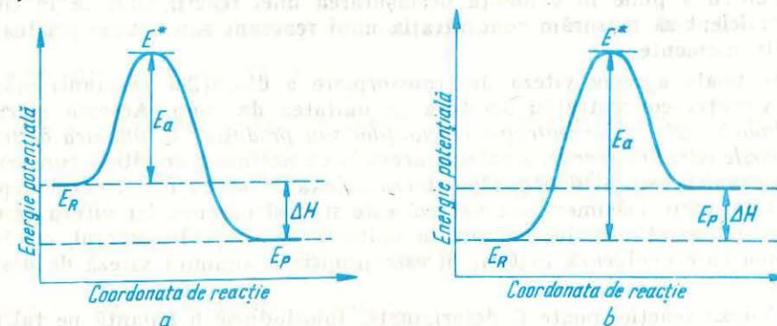
Fig. 3.6. Variația energiei potențiale în reacțiile chimice : a) \Delta H = E_p - E_r < 0 (r. exotermă) b) \Delta H = E_p - E_r > 0 (r. endotermă)
