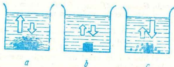
Fig. 4.3. Dizolvarea NaNO_3 : a — soluție nesaturată; b — soluție saturată; c — soluție suprasaturată.
