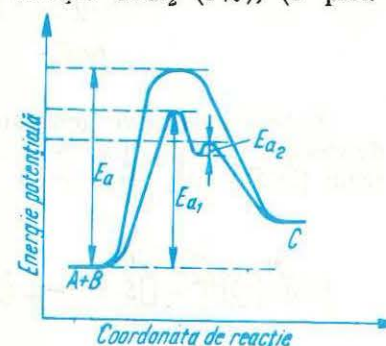
Fig. 3.22. Diagrama variației energiei potențiale pentru reacția în absența catalizatorului și în prezența catalizatorului.
