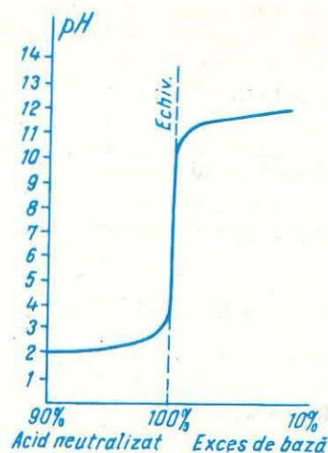
Fig. 4.11. Curba de neutralizare a unui acid tare cu o bază tare.
