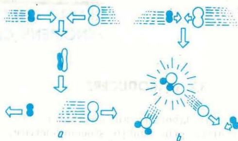
Fig. 3.2. Formarea complexului activat : a — reacția chimică nu are loc; b — reacția a avut loc.
