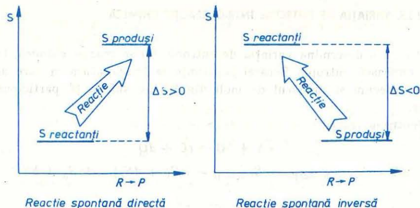
Fig. 2.12. Variația entropiei reacțiilor.
