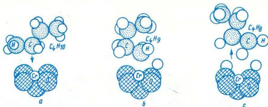
Fig. 3.31. Modelarea reacției de dehidrogenare a butanului: a — molecula de C_4H_{10} și catalizatorul; b — formarea C_4H_9\cdot și H\cdot ; c — formarea butenei.
