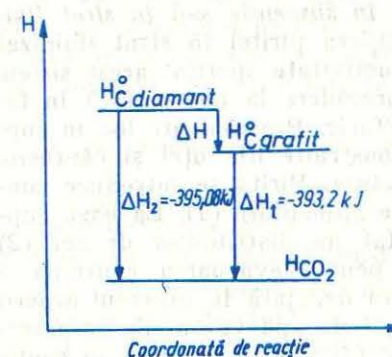
Fig. 2.7. Diagrama entalpiilor de reacție utilizată în calcularea entalpiei la transformarea C (diamant) în C (grafit).
