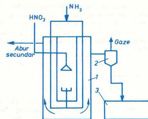
Fig. 2.10. Reactorul pentru obținerea azotatului de amoniu:
