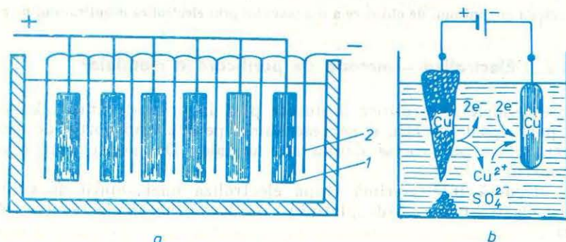
Fig. 1.15. Rafinarea cuprului :
