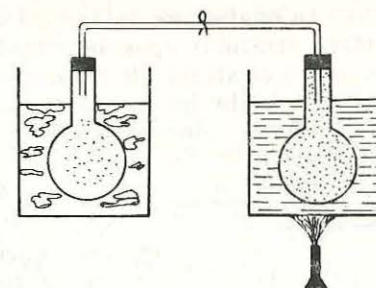
Fig. 4.5. Dispozitiv pentru verificarea influenței temperaturii asupra reacției de dimerizare a \text{NO}_2 .
