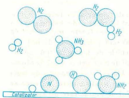
Fig. 3.29. Modelarea reacției de sinteză a amoniacului.
