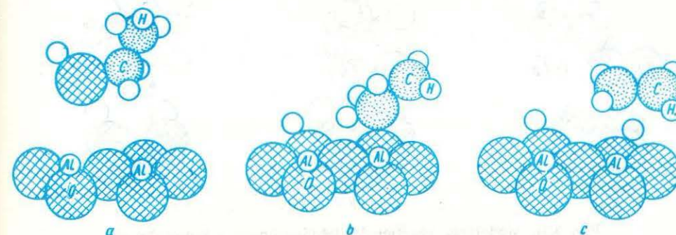
Fig. 3.30. Modelarea reacției de deshidratare a alcoolului etilic pe catalizator \text{Al}_2\text{O}_3 : a — molecula de alcool + catalizator; b — formarea ionului \text{C}_2\text{H}_5^+ fixat pe \text{O}^{2-} și \text{HO}^- pe \text{Al}^{3+} ; c — formarea etenei.
