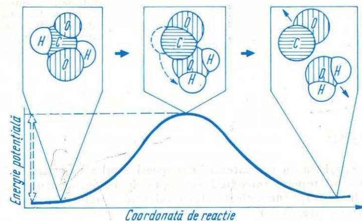
Fig. 3.23. Variația energiei potențiale pentru reacția de descompunere a acidului formic: \text{HCOOH} \rightarrow \text{CO} + \text{H}_2\text{O} .
