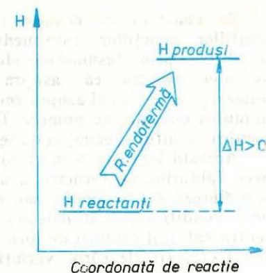
Fig. 2.5. Variația entalpiei de reacție în procesele endoterme.
