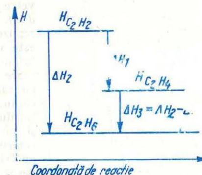
Fig. 2.8. Diagrama variației de entalpii de reacție, folosită pentru calculul entalpiei reacției de hidrogenare a etenei la etan.
