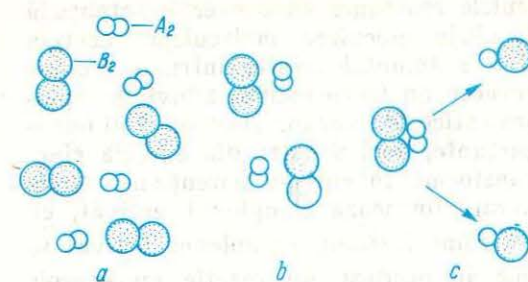
Fig. 3.4. Ciocnirea moleculelor A_2 și B_2 : a — orientare nefavorabilă; b — orientare favorabilă; c — formarea complexului activat și a produșilor de reacție.
