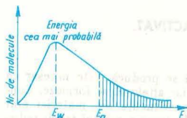
Fig. 3.3. Repartitia energiei între moleculele gazului.
