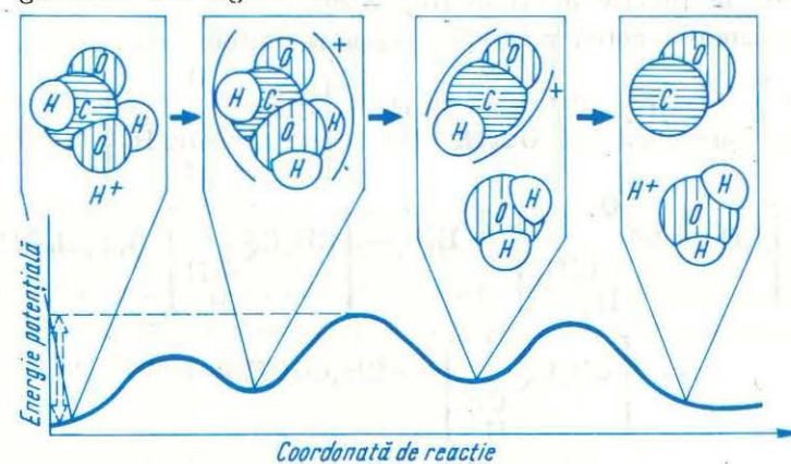
Fig. 3.24. Variația energiei potențiale pentru reacția de descompunere a acidului formic în prezența catalizatorului.
