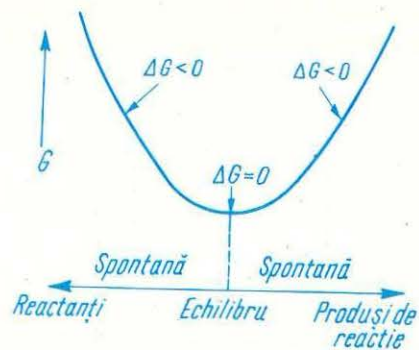
Fig. 4.2. Variația entalpiei libere pentru reacțiile chimice.
