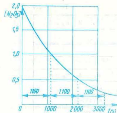
Fig. 3.15. Stabilirea timpului de înjumătățire prin metoda grafică pentru reacția de descompunere a N_2O_5 .
