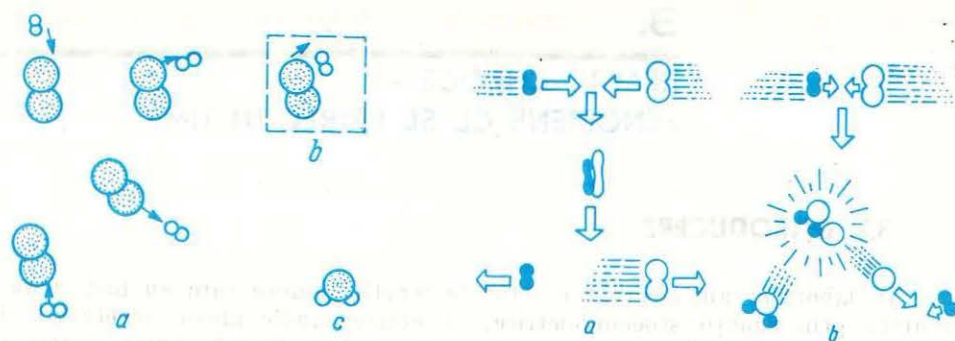
Fig. 3.1. Ciocniri între molecule : a — ciocniri neeficace; b — ciocniri eficiente; c — structura moleculei obținute.
