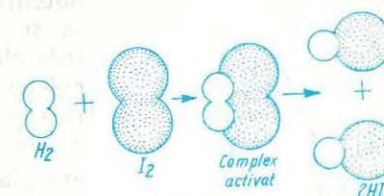
Fig. 3.5. Modelarea reacției chimice : H_2 + I_2 \rightarrow 2HI .
