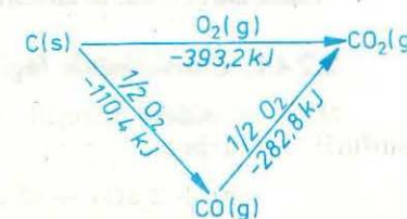
Fig. 2.6. Schema reacției de obținere a CO 2 .
