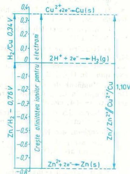
Fig. 1.7. Reprezentarea schematică a relației dintre valorile potențialelor normale de electrod pentru elementul galvanic Zn-Cu.
