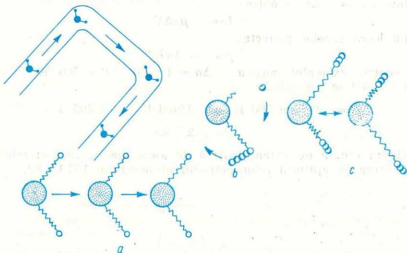
Fig. 2.2. Modelarea mișcării unei molecule de apă:
