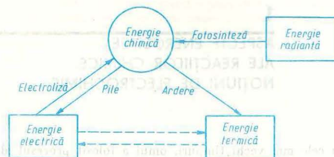
Fig. 1.1. Modalitățile de transformare a energiei chimice în alte forme de energie.
