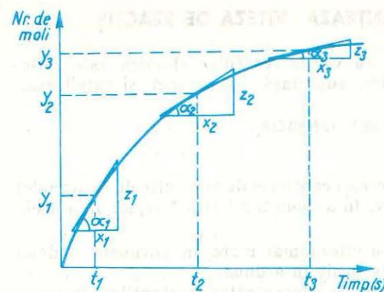
Fig. 3.10. Calculul vitezei de reacție prin metoda grafică.
