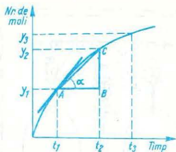
Fig. 3.9. Variația numărului de moli de \text{CO}_2 la diferite intervale de timp.
