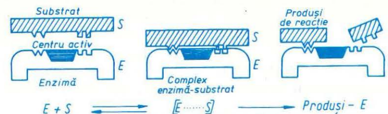
Fig. 3.32. Modelarea interacțiunii enzimului cu substratul.
