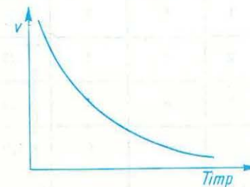
Fig. 3.12. Variația vitezei reacțiilor chimice în timp.
