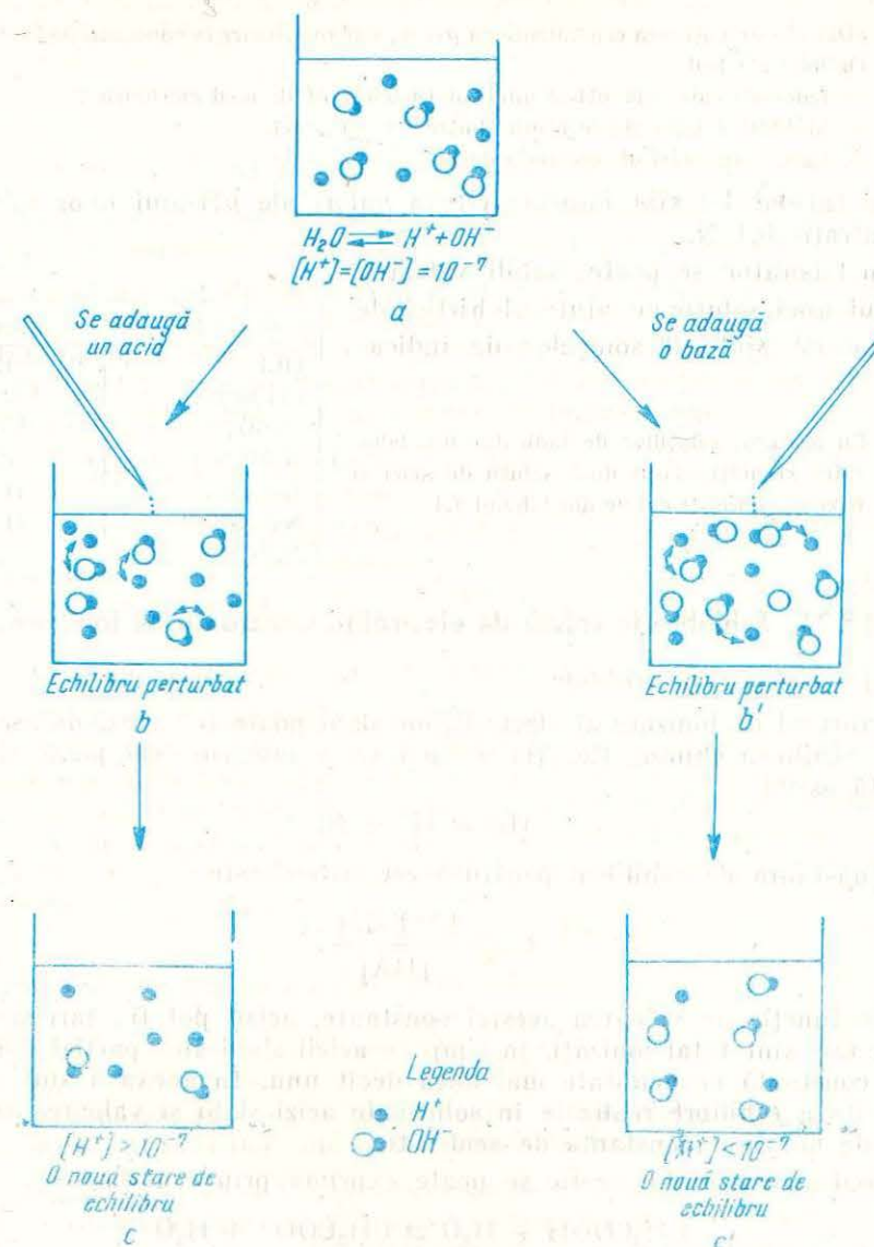
Fig. 4.10. Modelarea variației concentrației ionilor de hidrogen la adăugarea de acid și bază.
