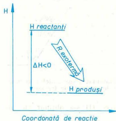
Fig. 2.4. Variația entalpiei de reacție în procesele exoterme.
