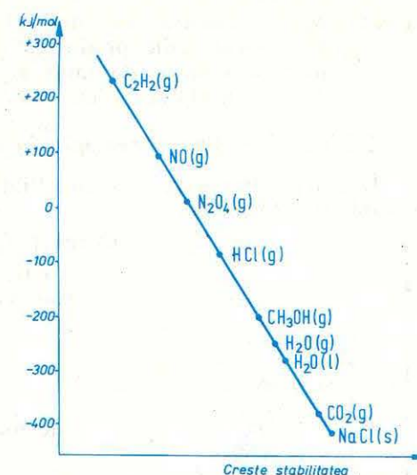
Fig. 2.3. Stabilitatea substanțelor în funcție de căldurile de formare.
