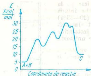
Fig. 3.17. Variația energiei potențiale pentru o reacție ce decurge în mai multe etape.
