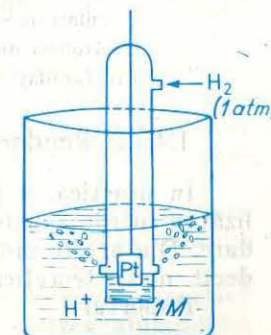
Fig. 1.5. Electrodul normal de hidrogen.
