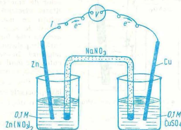
Fig. 1.3. Schema unui element galvanic.
