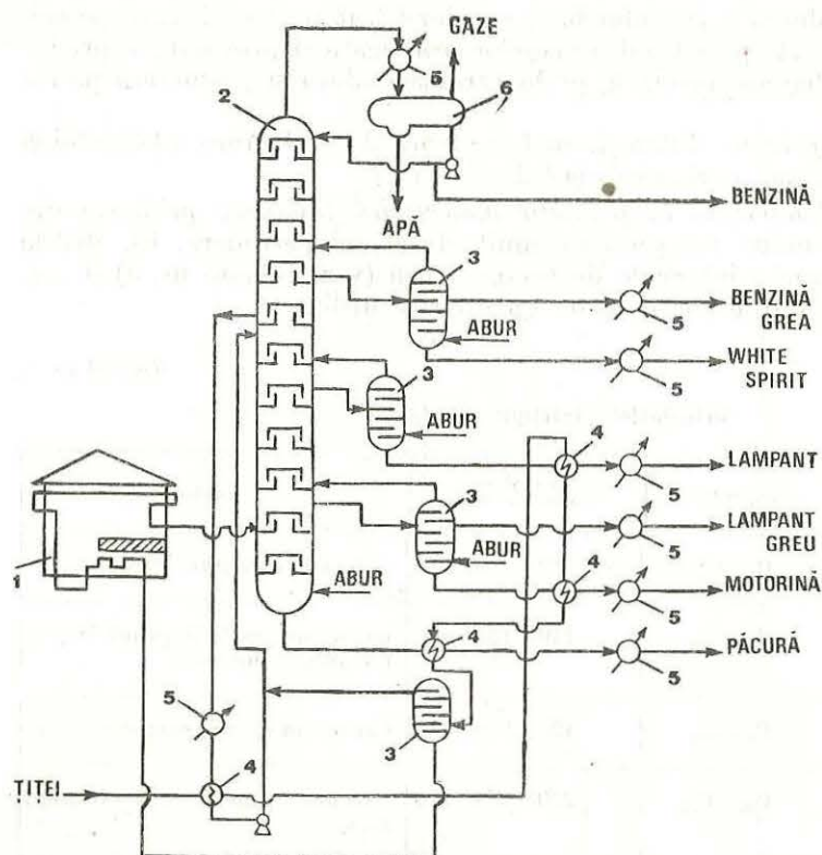
Fig. 24. Schema instalației de distilare primară:
