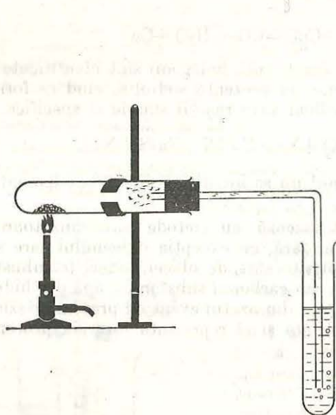
Fig. 5. Dispozitiv pentru identificarea carbonului și hidrogenului în compuşii organici.
