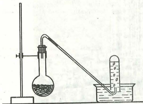
Fig. 18. Instalație de laborator pentru prepararea acetilenei din carbură de calciu.
