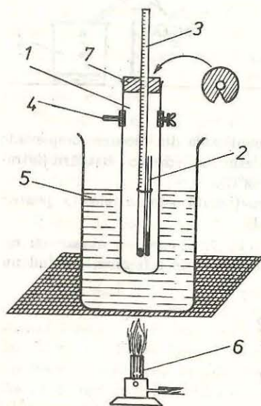
Fig. 4. Dispozitiv pentru determinarea punctului de topire:
