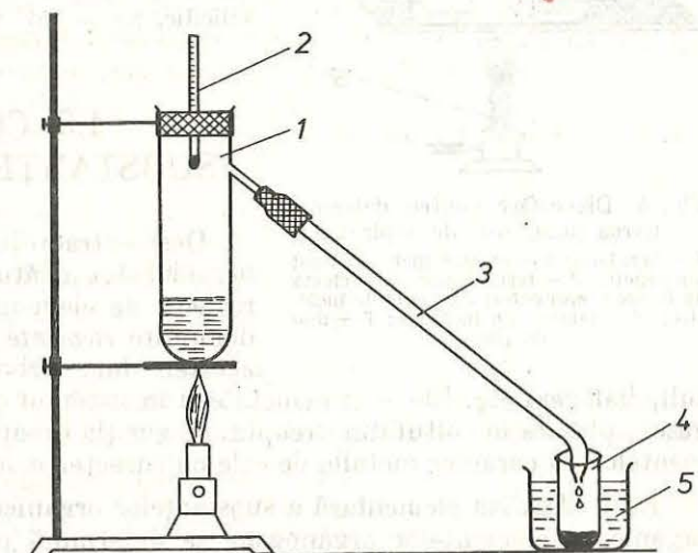
Fig. 3. Instalație de distilare fracționată simplă pentru cantități mici de substanțe:
