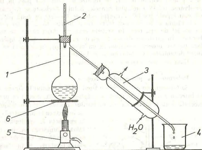
Fig. 2. Instalație de distilare fracționată simplă:
