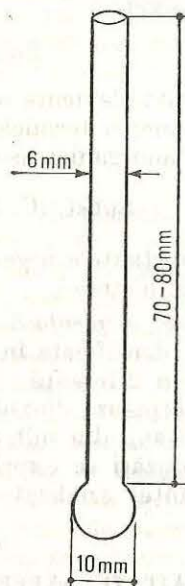
Fig. 6. Tubușor pentru mineralizarea compuşilor organici.
