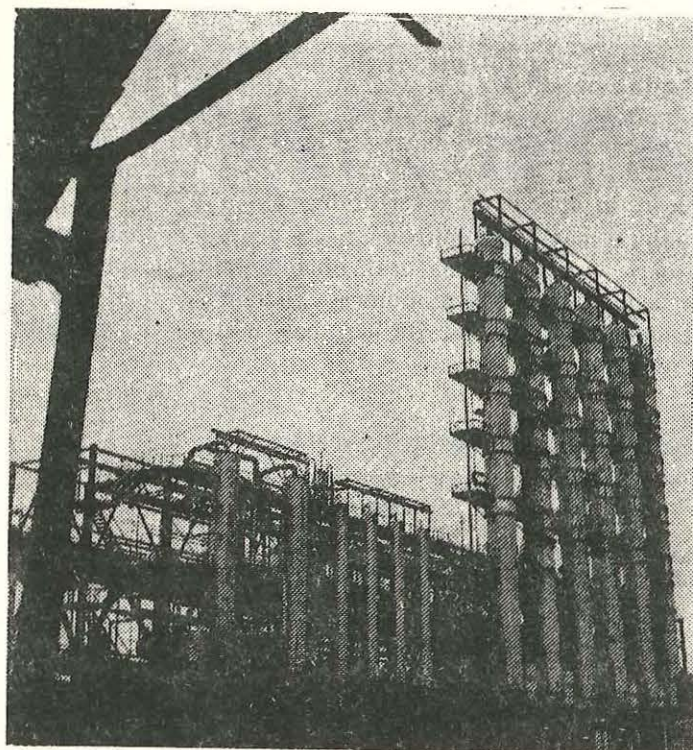
Secția de butadienă. Combinatul Petrochimic Borzești.
