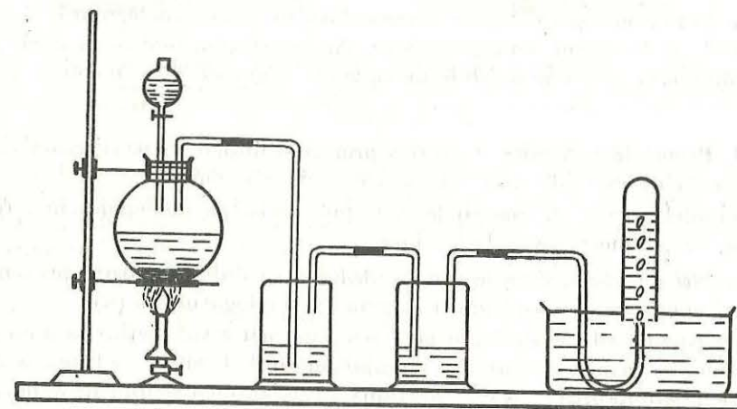
Fig. 15. Instalație de laborator pentru obținerea etenei din etanol și acid sulfuric.
