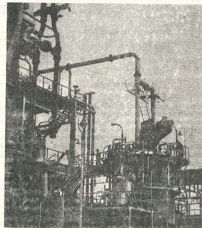
Combinatul Petrochimic Pitești. Instalația de polietenă de joasă presiune.
