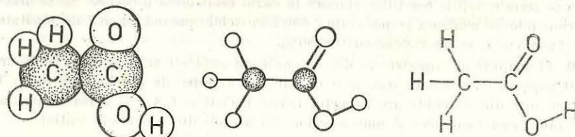
Fig. 31. Modelul spațial al moleculei de acid acetic (etanoic).
