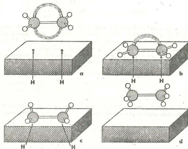
Fig. 16. Schema mecanismului hidrogenării catalitice a etenei: a) adsorbția hidrogenului la suprafața catalizatorului; b) adsorbția etenei la suprafața catalizatorului cu desfacerea dublei legături; c) adiția hidrogenului; d) desorbția etanului.
