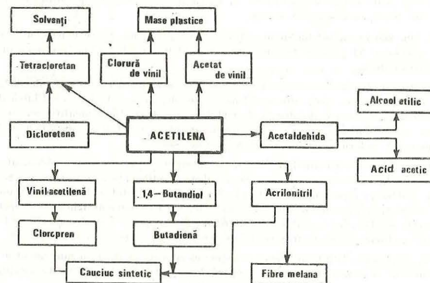
Fig. 20. Schema chimizării acetilenei.
