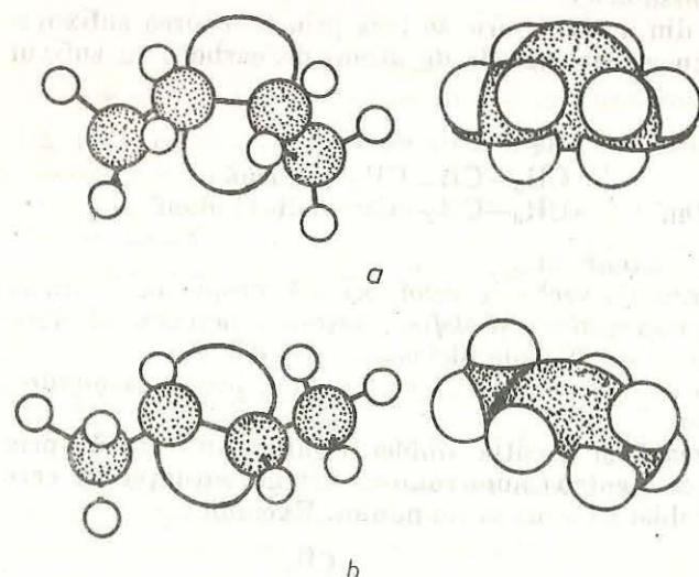
Fig. 14. Modelul spațial al izomerilor geometrici ai-2 butenei:
