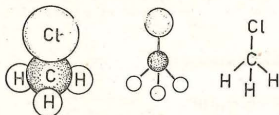
Fig. 25. Modelul spațial al moleculei de clormetan.
