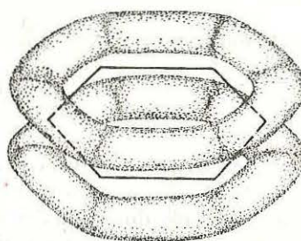
Fig. 22. Dispoziția primului orbital molecular la benzen.
