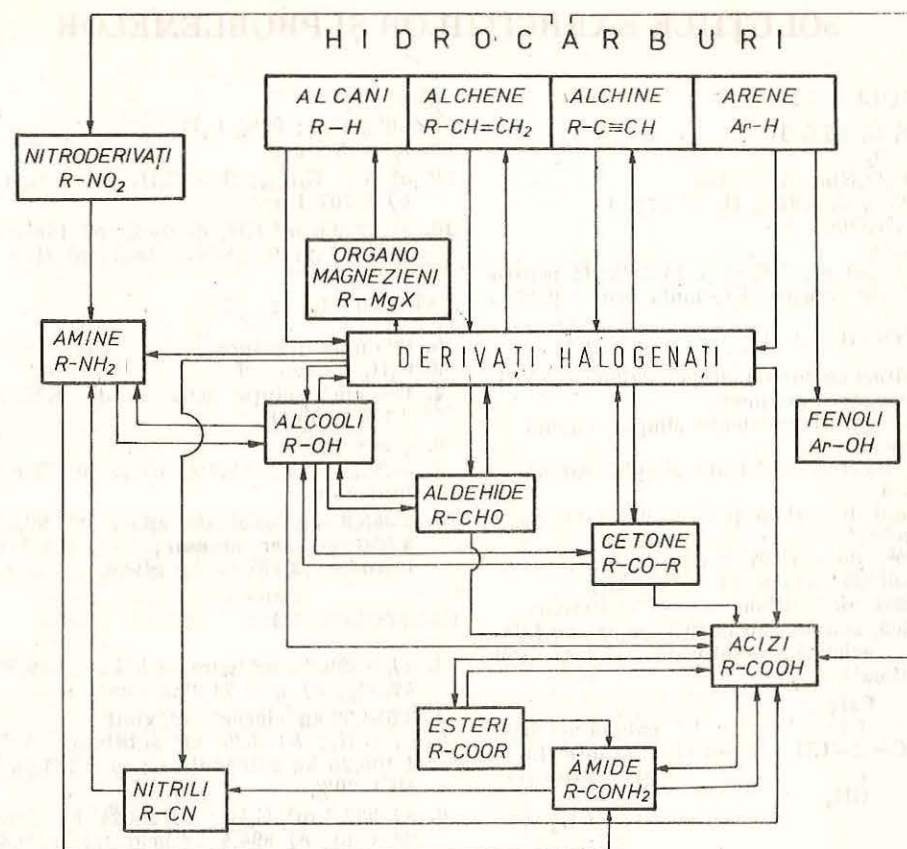
Fig. 36. Schema relațiilor dintre diferitele clase de compuși organici.
