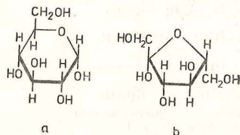
Fig. 32. Formulele de perspectivă ale glucozei (a) și fructozei (b).
