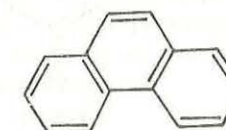
fenantren
