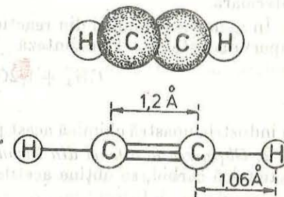
Fig. 17. Modelul spațial al moleculei de acetilenă.
