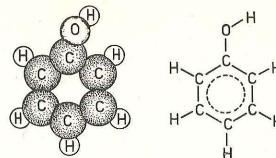
Fig. 27. Modelul spațial al moleculei de fenol.
