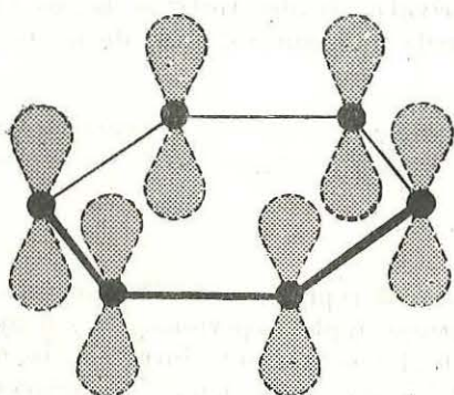
Fig. 21. Dispoziția spațială a orbitalilor atomici în ciclul benzenic.
