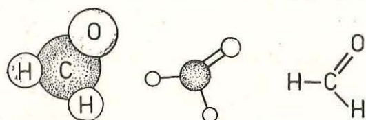
Fig. 28. Modelul spațial al moleculei de aldehydă formică (metanal).
