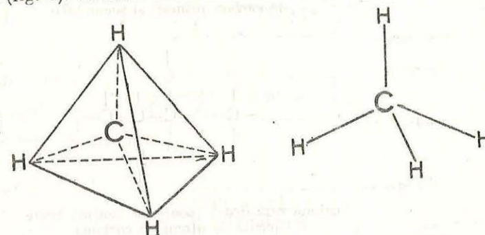
Fig. 7. Structura tetraedrică a moleculei de metan, \text{CH}_4 .
