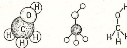
Fig. 26. Modelul spațial al moleculei de alcool metilic.
