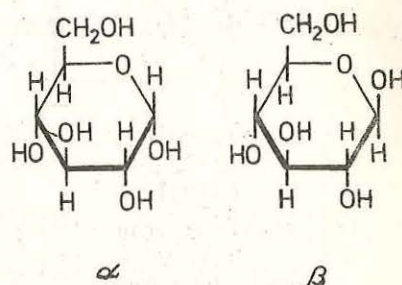
Fig. 33. Formulele de perspectivă ale α- și β-glucozei.
