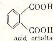
acid ortoftalic
