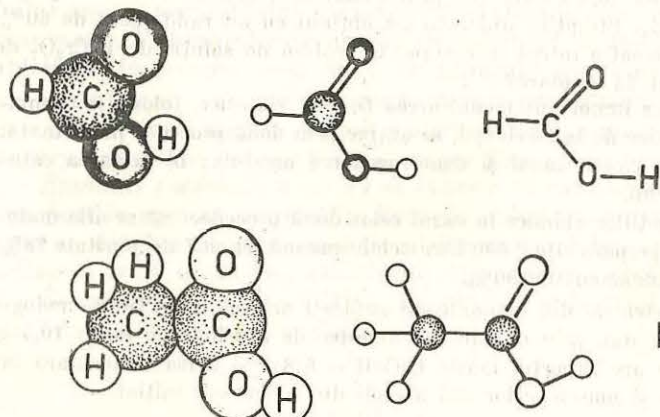
Fig. 31. Modelul spațial al moleculei de acid acetic (etanoic).
