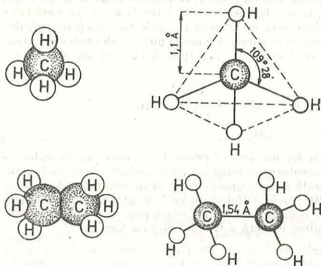
Fig. 9. Modelele spațiale ale moleculelor de metan și de etan.
