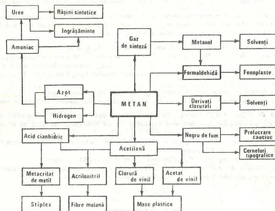
Fig. 12. Schema chimizării metanului.
