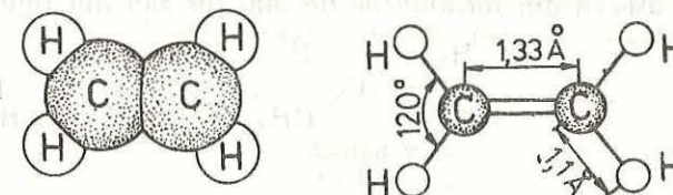
Fig. 13. Modelul spațial al moleculei de etenă.
