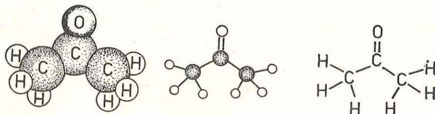
Fig. 29. Modelul spațial al moleculei de acetona (propanonă).
