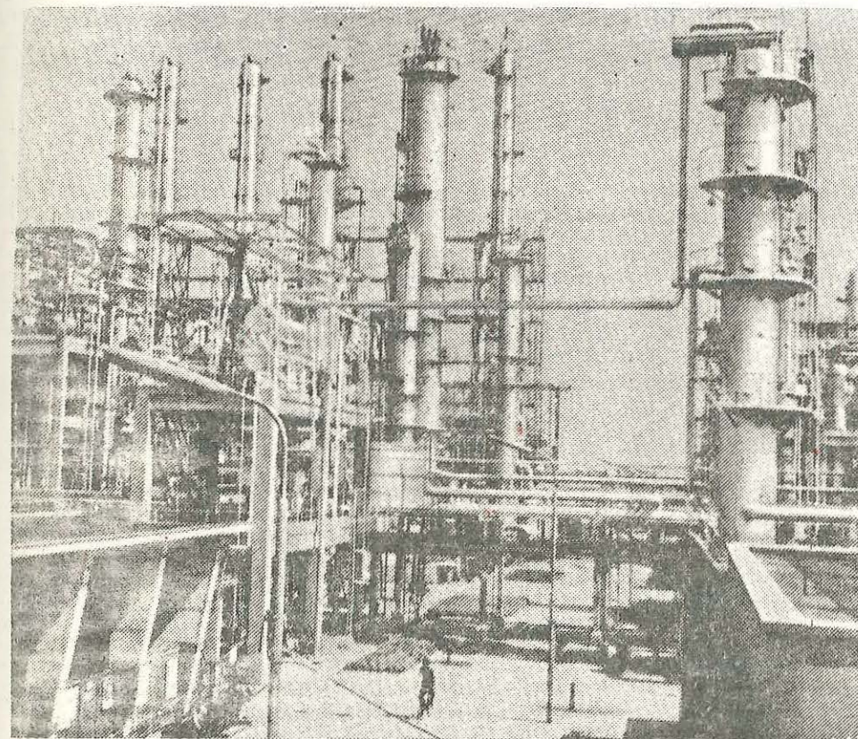
Instalație de reformare catalitică. Combinatul Petrochimic Brazi.
