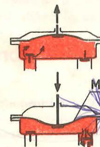
Fig. 2.127. Pompa de benzină.
