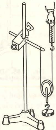
Fig. 2.55. Dispozitiv pentru studiul forțelor la scripetele mobil.
