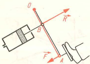
Fig. 2.45. Pedala de frână a unui automobil este o pîrghie cu punctul de sprijin la un capăt și forța activă la celălalt.
