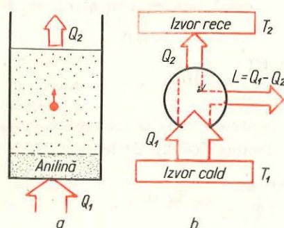
Fig. 4.8. Principiul motorului termic. a) Anilina se mișcă atunci când vasul este încălzit. b) Schema principiului motorului termic.
