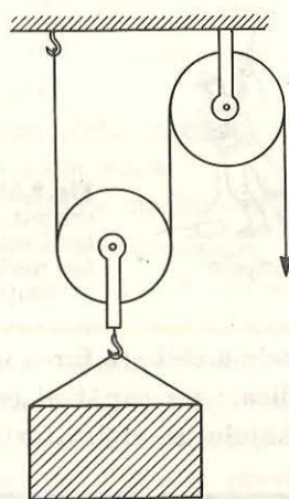
Fig. 2.56. Scripete compus.
