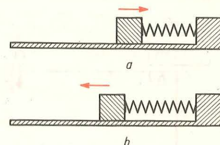
Fig. 2.65. Sistem fizic alcătuit dintr-un corp care ciocnește un resort: a) în timpul comprimării resortului energia cinetică se transformă în energie potențială; b) prin destinderea resortului energia potențială se transformă în energie cinetică.
