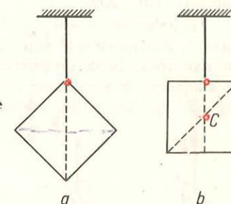
Fig. 2.82. Determinarea experimentală a centrului de greutate al unei plăci.
