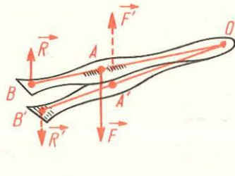
Fig. 2.46. Penseta este un ansamblu de două pîrghii, cu punctul de sprijin la un capăt și forța rezistentă la celălalt capăt.
