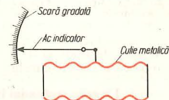
Fig. 2.113. Barometrul metalic.
