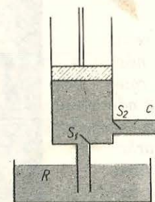
Fig. 2.123. Pompă aspiro-respingătoare.
