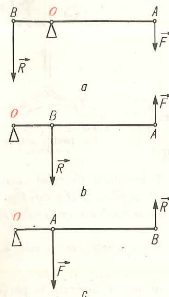
Fig. 2.40. Poziția punctului de sprijin la o pîrghie: a) între punctul de aplicație al forței active și cel al forței rezistente; b) la un capăt al pîrghiei, la celălalt capăt fiind punctul de aplicație al forței active; c) la un capăt al pîrghiei, la celălalt capăt fiind punctul de aplicație al forței rezistente.
