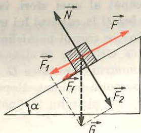
Fig. 2.60. Forțele ce se exercită asupra corpului care urcă uniform, cu frecare, pe planul înclinat.
