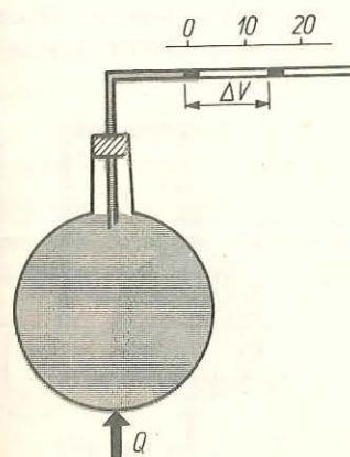
Fig. 4.3. Dispozitiv experimental pentru studiul dilatării gazelor la presiune constantă.
