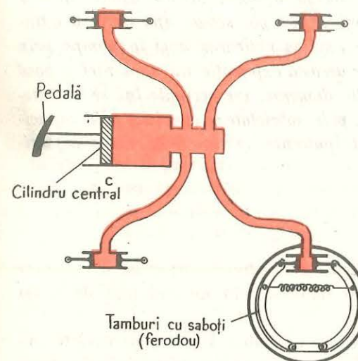
Fig. 2.109. Schema frînei hidraulice.
