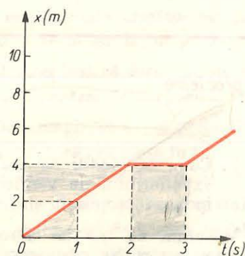
Fig. 1.1. Graficul mișcării primului mobil din problema 11.
