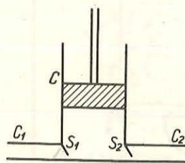
Fig. 2.120. Pompă pentru gaze.
