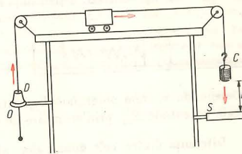
Fig. 2.61. Dispozitiv pentru studiul lucrului mecanic efectuat de un corp în mișcare.
