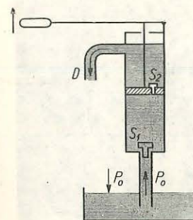
Fig. 2.122. Pompă aspiratoare.
