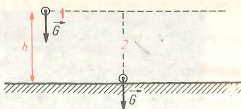
Fig. 2.63. Sistemul corp-Pământ în două stări diferite.
