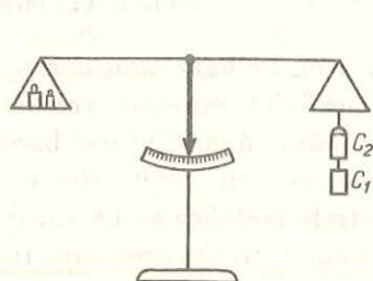
Fig. 2.115. Balanță cu cilindrii lui Arhimede în echilibru.
