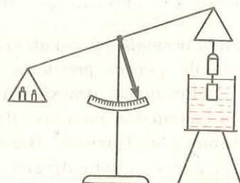
Fig. 2.116. Balanța dezechilibrată datorită forței arhimedice.
