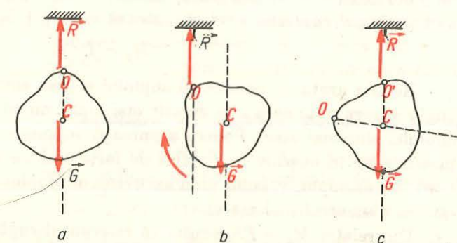
Fig. 2.81. Echilibrul unui corp suspendat: a) la echilibru greutatea și reacțiunea în fir sînt pe aceeași verticală; b) în caz contrar, brațul cuplului este diferit de zero și corpul se rotește; c) schimbînd punctul de susținere în O' , la echilibru O' și C sînt pe aceeași verticală.
