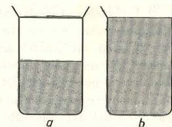
Fig. 5.3. Difuziunea lichidelor.
