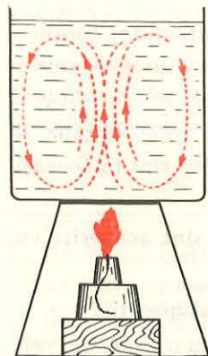
Fig. 4.11. Convecția în lichide.
