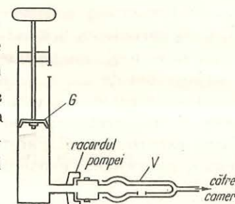
Fig. 2.121. Pompa de bicicletă.
