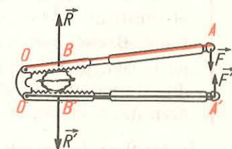
Fig. 2.44. Cleștele de spart nuci este un ansamblu de două pîrghii cu punctul de sprijin la un capăt și forța activă la celălalt.
