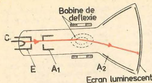
Fig. 1.14. Tub cinescop.
