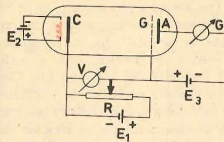
Fig. 2.10. Schema dispozitivului Franck și Hertz. E_1 — sursa tensiunii de accelerare a electronilor, E_2 — sursa tensiunii de încălzire a filamentului, E_3 — sursa de tensiune pentru cimpul contrar, între anodul A și grila G.
