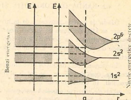
Fig. 3.19. Formarea benzilor energetice din nivelele energetice discrete ale atomilor ( a este constanta rețelei cristaline).
