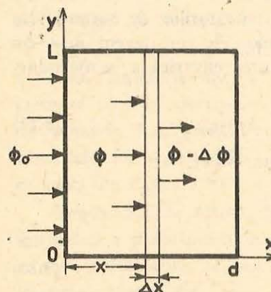
Fig. 3.27. Absorbția luminii într-un semiconductor cu grosimea d și înălțimea L .
