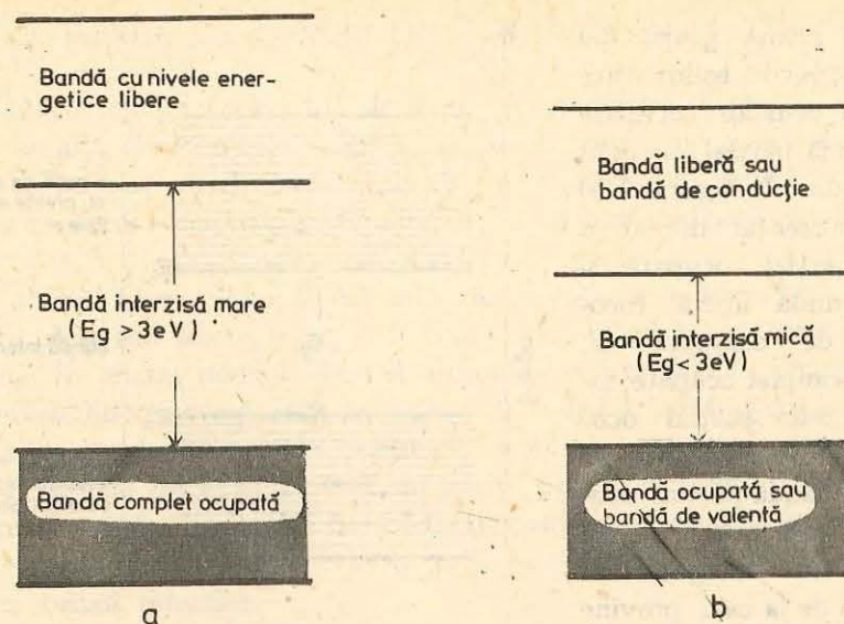
Fig. 3.22. Reprezentarea schematică a benzilor energetice în cazul izolatoarelor (a) și în cazul semiconductorilor (b).
