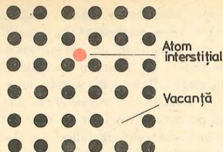
Fig. 3.6. Modelul bidimensional al unei rețele de atomi cu defecte punctiforme.
