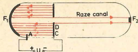
Fig. 1.19. Producerea razelor canal: A — anod, C — catod, D — orificiu în catod, F_1 și F_2 — luminescența sticlei.
