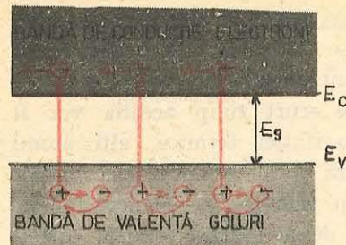
Fig. 3.24. Reprezentarea schematică a principalelor procese fizice care au loc într-un semiconductor cu conducție intrinsecă.
