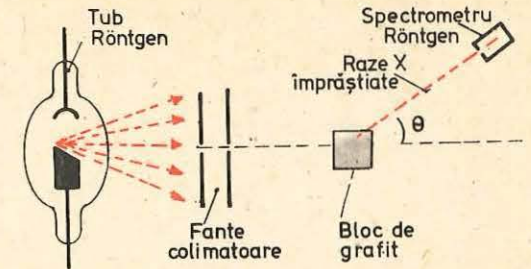
Fig. 1.15. Schema experienței pentru efectul Compton.
