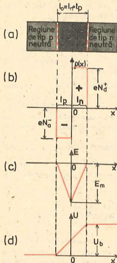
Fig. 3.32. Reprezentarea schematică a sarcinilor electrice din stratul de baraj al unei joncțiuni p-n , a ); distribuția densității de sarcină, b ); a câmpului electric, c ) și a potențialului, d ). Mărimea I_0 reprezintă lărgimea regiunii de sarcină spațială în absența polarizării.
