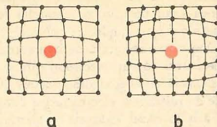
Fig. 3.7. Deformarea rețelei cristaline plane în cazul cind atomul impurității interstițiale a) sau substituționale b) are dimensiuni mai mari decît atomii de bază ai rețelei.
