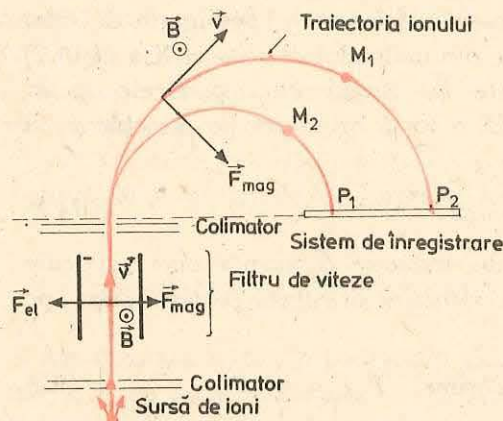
Fig. 4.1. Schema de principiu a unui spectrograf de mase. Traiectoria ionului de masă M_1 va avea raza mai mare decât cea a ionului de masă M_2 , dacă sarcina și viteza lor sunt aceleași dar M_1 > M_2 .
