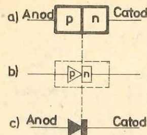
Fig. 3.34. Dioda semiconductor: a) reprezentarea schematică a unei joncțiuni p-n ; b) forma celor două materiale astfel modelată încât să corespundă sensului direct al curentului; c) simbolul diodei.
