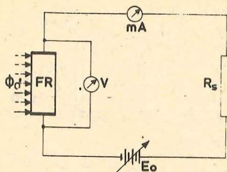
Fig. 3.30. Schema circuitului electric pentru studierea fotoconducției în semiconductori. Fotorezistența (FR) este conectată în serie cu o sursă de tensiune E_0 , rezistența de sarcină R_s și un miliampermetru. Căderea de tensiune pe fotorezistență se măsoară cu voltmetrul V .
