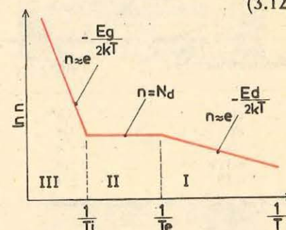
Fig. 3.26. Influența temperaturii asupra concentrației purtătorilor de sarcină într-un semiconductor electronic: I — regiunea cu conducție de impurități; II — regiunea de epuizare; III — regiunea de conducție intrinsecă.
