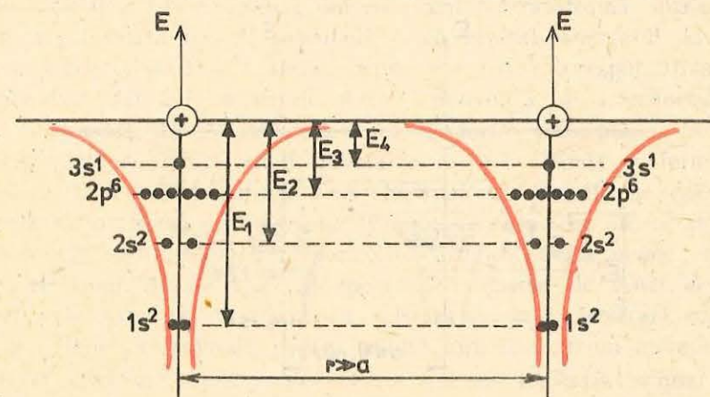
Fig. 3.17. Reprezentarea schematică a nivelelor energetice în cazul a doi atomi de Na aflați la o distanță r mult mai mare decît distanța interatomică a din cristalul de Na. Mărimilor E_1 , E_2 , E_3 și E_4 le corespund barierele de potențial pe care trebuie să le depășească un electron care se află pe nivelul energetic corespunzător pentru a părăsi atomul de care aparține.
