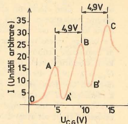
Fig. 2.11. Diagrama curent-tensiune în experiența Franck și Hertz cu vapori de mercur. I — intensitatea curentului prin galvanometru Gv. U_{CG} — tensiunea de accelerare catod-grilă; tensiunea retardantă U_{AG} = 0,5 \text{ V} , presiunea vaporilor de mercur p = 1 \text{ Torr} .
