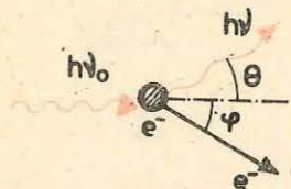
Fig. 1.16. Fotonul împrăștiat și electronul de recul în efectul Compton.
