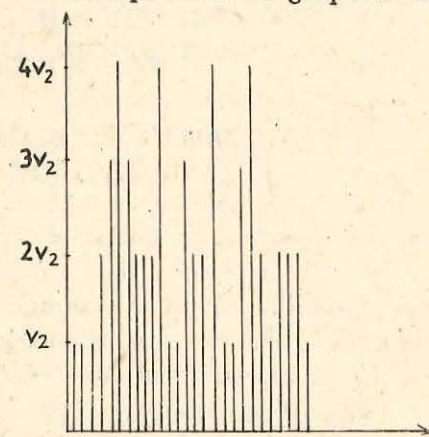
Fig. 1.26. Diagrama vitezelor picăturilor.
