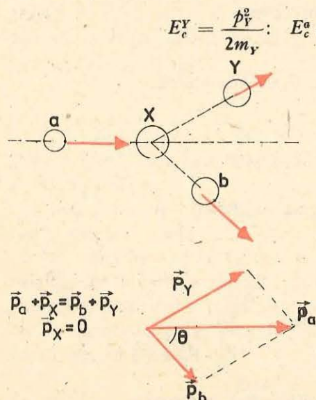
Fig. 4.6. Conservarea impulsului în reacția nucleară: a + X \rightarrow b + Y .
