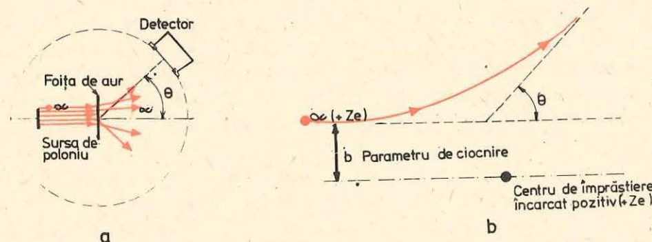
Fig. 2.2. a) Experiența de împrăștiere a particulelor \alpha efectuată de Rutherford. Particulele \alpha emise de sursa de poloniu sînt împrăștiate de foița de aur. Detectorul poate înregistra particule \alpha împrăștiate de foița de aur la orice unghi \theta , deoarece el se poate roti în jurul unei axe perpendiculare pe figură, în centrul dispozitivului. Sursa și foița se mențin în poziție fixă, legate de axă. b) Traectoria unei particule \alpha în cîmpul de forțe electrostatice de respingere creat de o particulă încărcată pozitiv ( Ze ); \theta este unghiul de împrăștiere.
