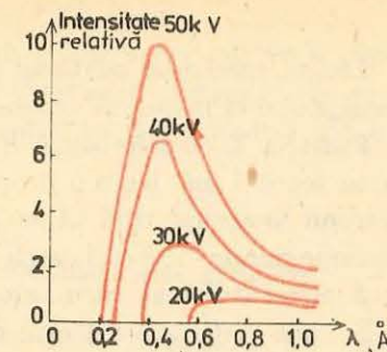
Fig. 2.21. Spectrul radiației X de frinare pentru diferite valori ale potențialului de accelerare. Spectrul începe de la o lungime de undă minimă care corespunde energiei maxime a radiației de frinare: h\nu_{max} = eU .
