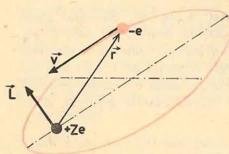
Fig. 2.12. Mișcarea unui electron pe o orbită eliptică. Momentul cinetic \vec{L} este perpendicular pe \vec{r} și \vec{v} deci perpendicular pe planul orbitei. Forța de atracție acționează pe direcția razei vektore \vec{r} .
