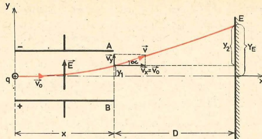
Fig. 1.20. Deviația unei particule încărcate pozitiv aflată în cîmp electric uniform, \vec{E} ; A și B — armăturile condensatorului plan.
