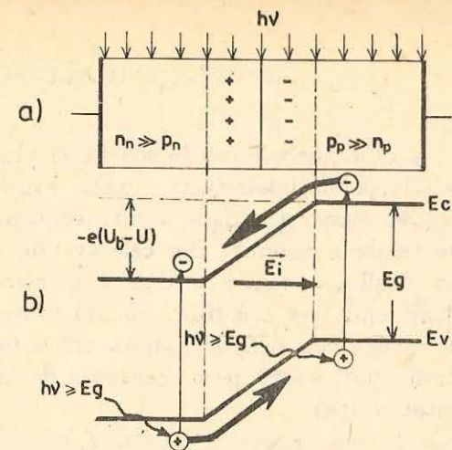
Fig. 3.35. Reprezentarea schematică a unei joncțiuni p-n (a) și structura energetică în prezența iluminării (b).
