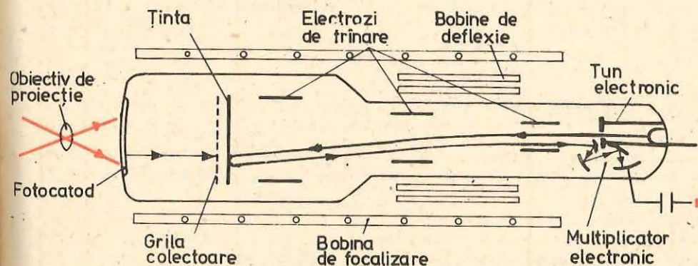
Fig. 1.13. Tub videocaptor.
