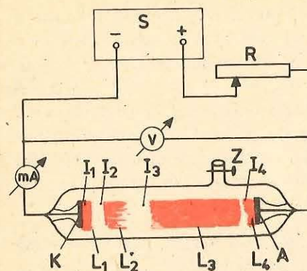
Fig. 5.3. Descărcarea luminescentă în curent continuu.
