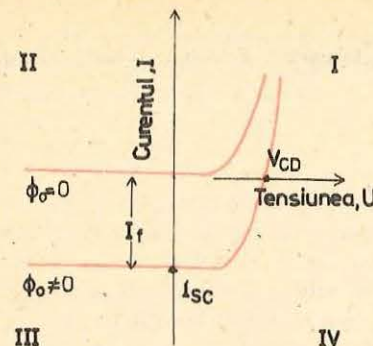
Fig. 3.36. Caracteristica curent-tensiune a unei joncțiuni p-n în absența și în prezența iluminării ( \Phi_0 = 0 , respectiv \Phi_0 \neq 0 ).
