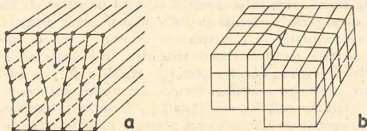
Fig. 3.8. Două tipuri de dislocații într-o rețea de atomi; a) dislocația marginală; b) dislocația în spirală.
