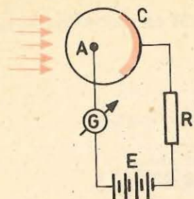
Fig. 1.7. Celula fotoelectrică.
