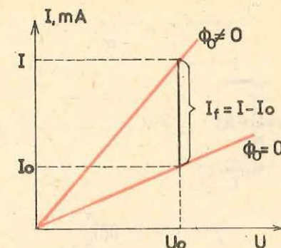
Fig. 3.29. Caracteristica curent-tensiune a unei fotorezistențe în absența ( \Phi_0 = 0 ) și în prezența iluminării ( \Phi_0 \neq 0 ).
