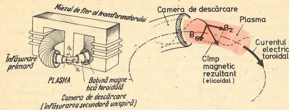
Fig. 5.12. Formarea configurației de câmp magnetic elicoïdal în instalația TOKAMAK.
