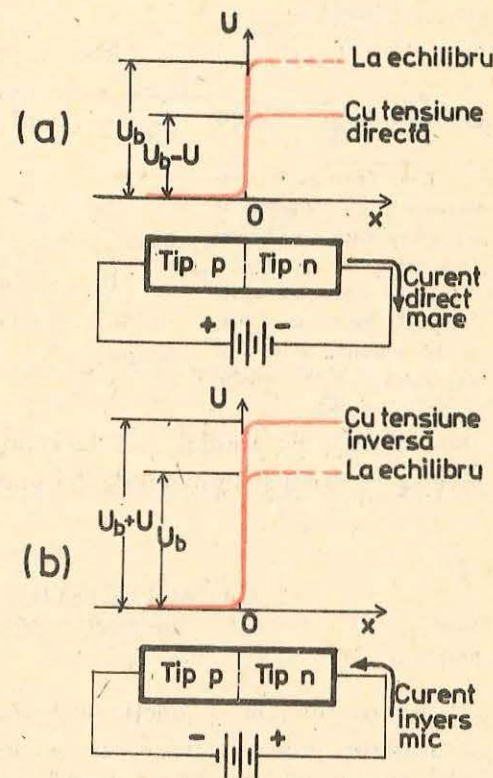
Fig. 3.33. Polarizarea directă a ) și polarizarea inversă b ) a unei joncțiuni p-n .
