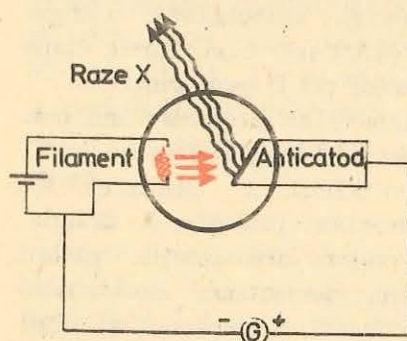
Fig. 2.19. Tubul de raze X. Electronii emiși de un filament încălzit sînt accelerați de câmpul electric dintre catod (filament) și anod (anticatod). În urma ciocnirii acestora cu anticatodul iau naștere radiații X.
