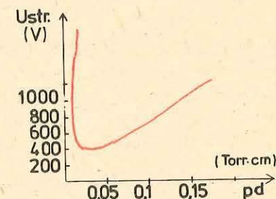
Fig. 5.4. Curba Paschen în aer, cu electrozi de fier.
