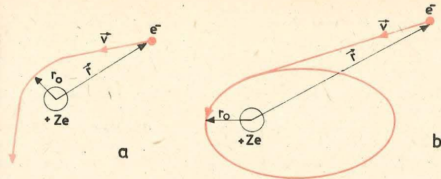
Fig. 2.4. Traietoriile unui electron care se mișcă în jurul nucleului încărcat pozitiv: a) trajectorie deschisă, stare liberă; b) trajectorie închisă, stare legată; r_0 este distanța cea mai mică la care se poate apropia electronul de nucleul încărcat pozitiv, pentru o anumită energie cinetică inițială.
