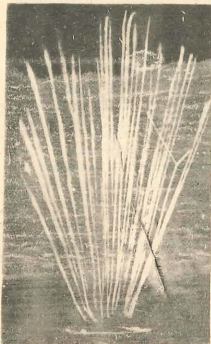
Fig. 4.19. Dezintegrări fotografiate în camera cu ceață.
