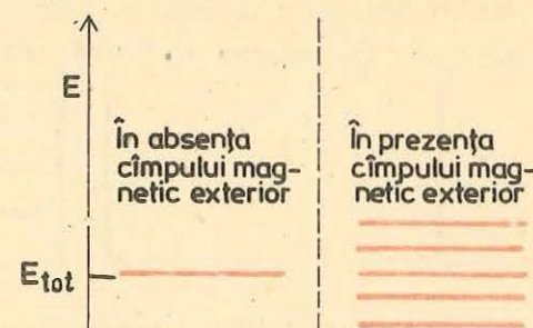
Fig. 2.15. Modificarea energiei totale a electronului în prezența câmpului magnetic în cazul în care numărul cuantic orbital are valoarea l=2 . În locul unui singur nivel, apar 2l+1=5 subnivele.
