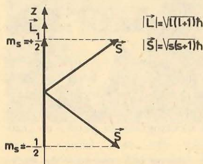
Fig. 2.17. Orientarea momentului cinetic de spin în cîmpul magnetic creat de momentul cinetic orbital.
