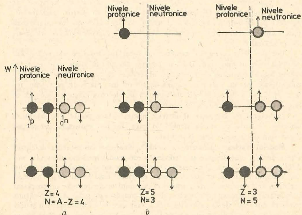
Fig. 4.4. Așezarea nucleonilor în modelul păturilor nucleare. Nucleul cu A=8 este cel mai stabil în configurația a ) în care păturile sunt ocupate. În configurațiile b ) și c ) în care există un surplus de protoni sau de neutroni, nucleonul suplimentar se așază pe o pătură cu energie de legătură mai mică. Protonul a fost reprezentat ca un cerc de culoare închisă iar neutronul ca un cerc hașurat. Săgeata indică orientarea momentului cinetic de spin.
