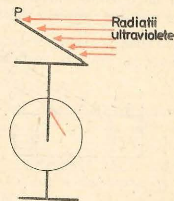
Fig. 1.1. Punerea în evidență a efectului fotoelectric extern pe suprafața metalică P cu ajutorul electrosopului.
