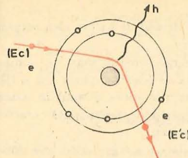
Fig. 2.20. Producerea radiației X de frinare de către un electron în câmpul electrostatic al nucleului.
