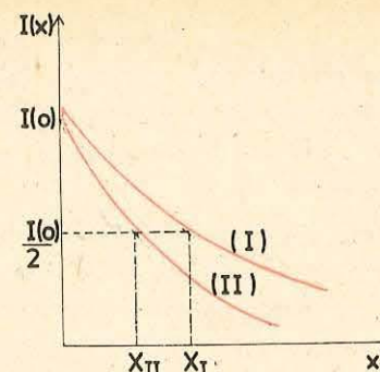
Fig. 4.14. Variația intensității de radiații cu grosimea stratului de substanță străbătut pentru două cazuri: (I) substanță cu coeficient de atenuare mic; (II) substanță cu coeficient de atenuare mare. X_I și X_{II} reprezintă grosimile de înjumătățire în cele două cazuri.
