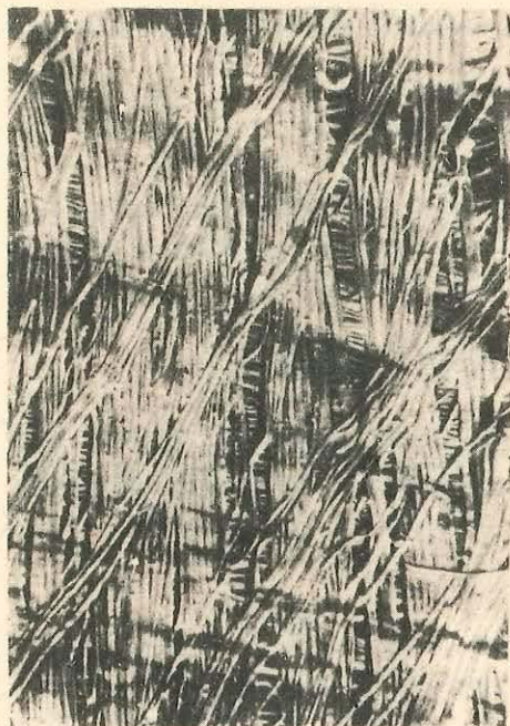
Fig. 1.31. Secțiune prin fibra nervoasă; imagine obținută cu microscopul electronic.
