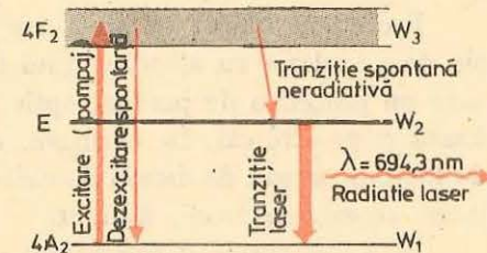
Fig. 2.24. Nivele energetice ale ionului de Cr^{+++} implicate în emisia laser a cristallului de rubin (laser cu trei nivele).
