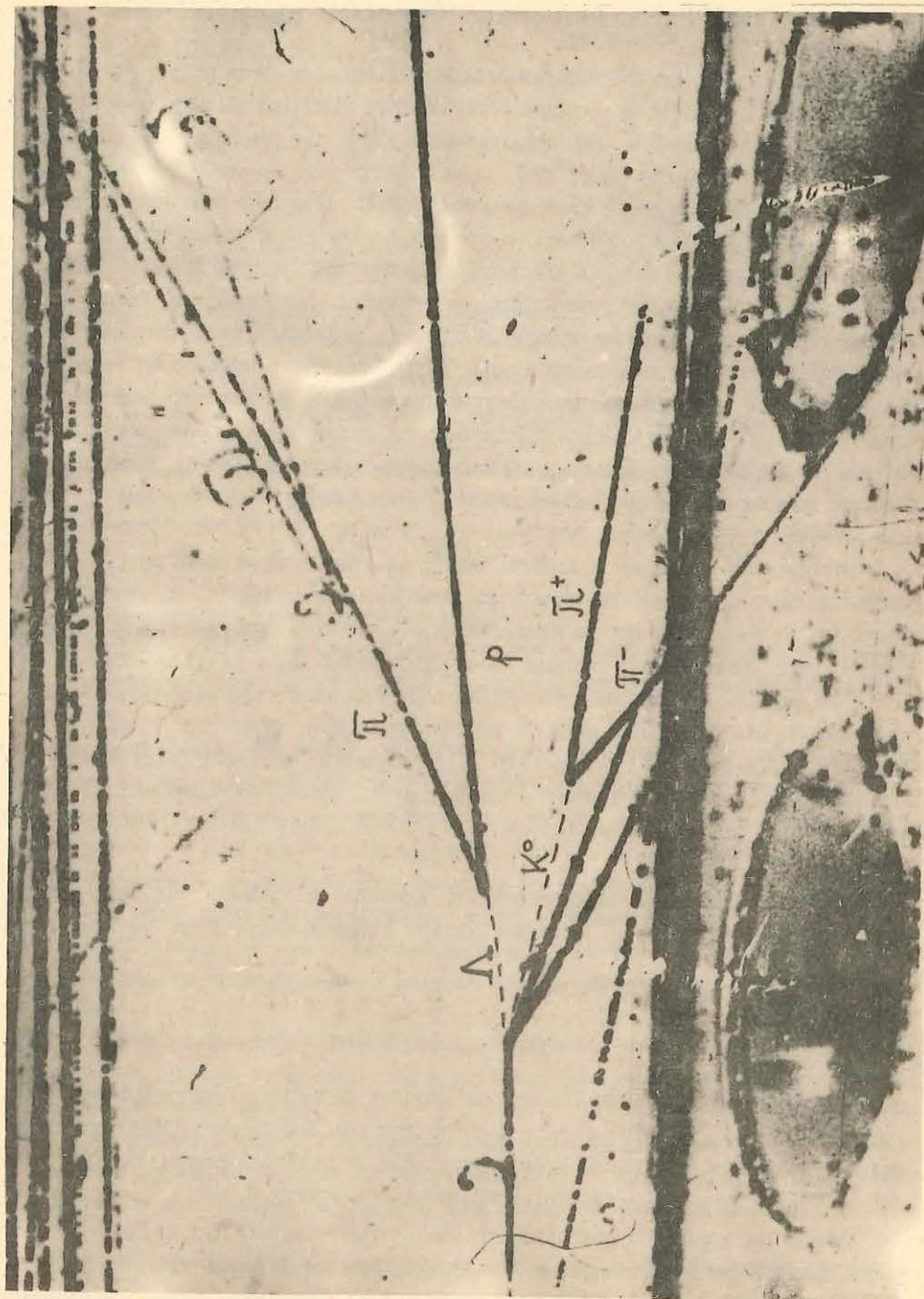
Fig. 4.24. Generare de perechi.
