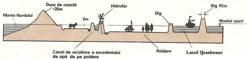
Fig. 42. Secțiune prin terenurile asanate de la mare.
