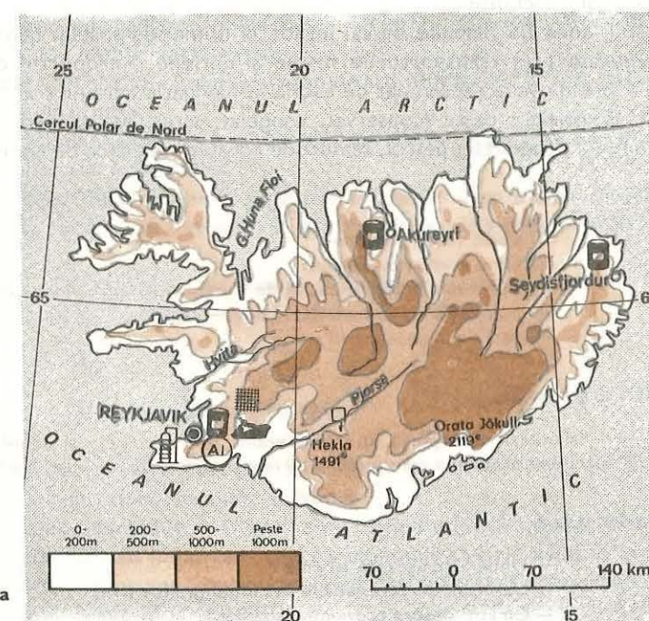
Fig. 72. Islanda — Harta fizică și economică
