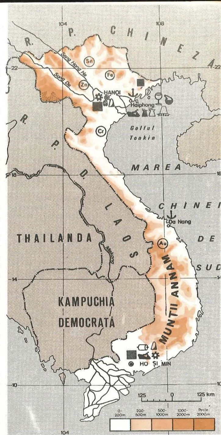
Fig. 99. R.S. Vietnam — Harta fizică și economică
