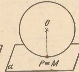
OP = OM = R
