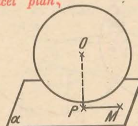
R < OP < OM
