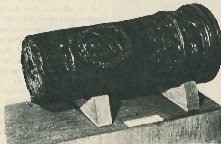
Tun din sec. al XVI-lea pe care se vede stema Țării Românești
