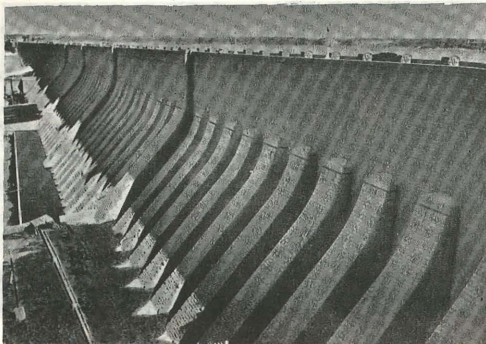
Marele baraj de la Assuan.
