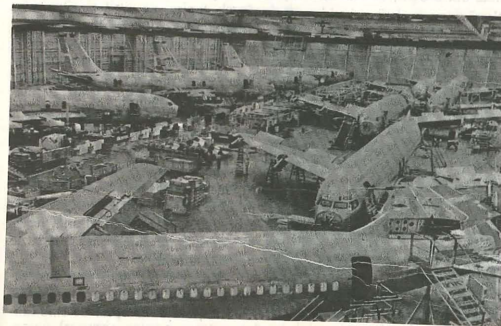
Atelier de montaj într-o uzină de avioane în S.U.A.
