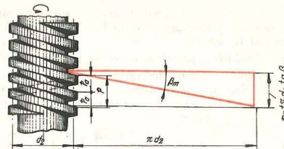
Fig. 9.9. Elicea cilindrică a filetelui desfășurat.
