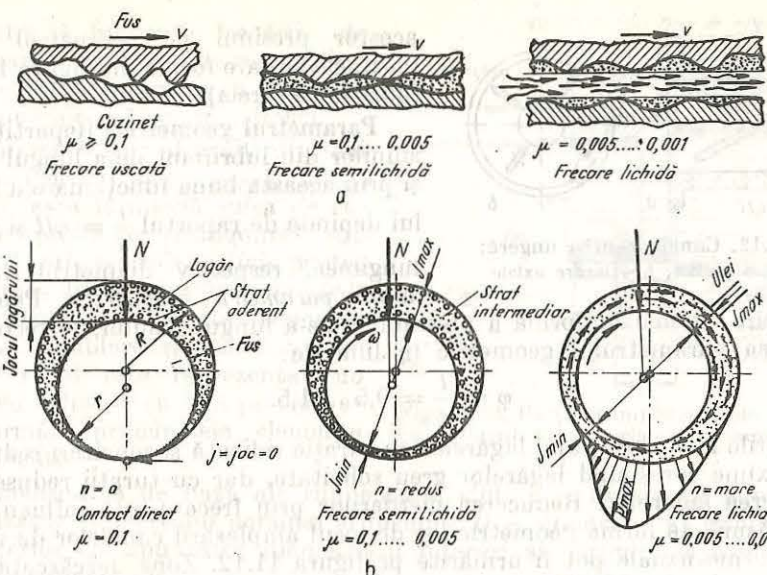
Fig. 11.11. Frecarea în lagăre:
