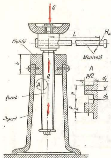
Fig. 9.14. Cric cu șurub-piuliță pentru transmisia forțelor: Q — forța de lucru; Q_m — forța de acționare la manivelă.
