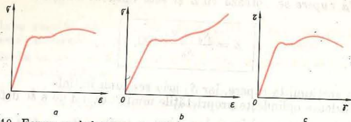
Fig. 1.10. Forma curbelor caracteristice ale oțelului moale la diverse solicitări: a — la întindere și încovoiere; b — la compresiune; c — la răsucire.
