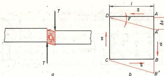
Fig. 3.2. Deformația la forfecare.
