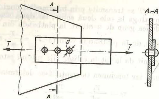
Fig. 3.5. Nituirea a două piese prin suprapunere.
