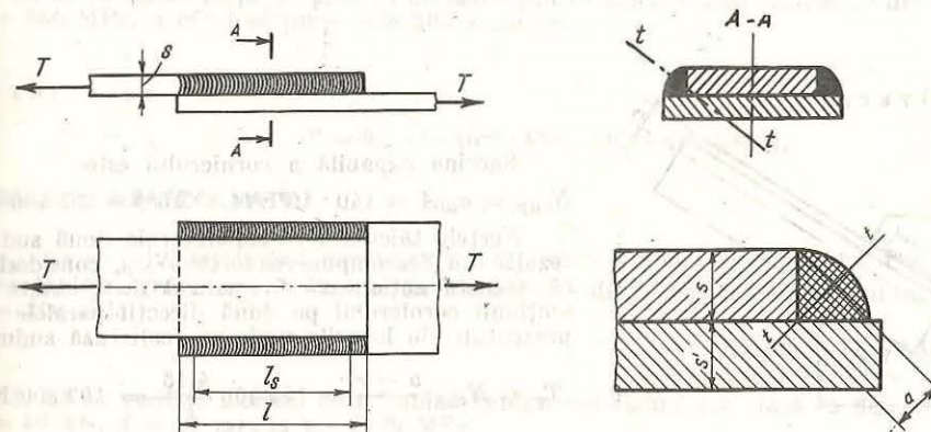
Fig. 3.7. Asamblare sudată.
