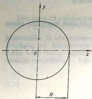
Fig. 4.4. Determinarea momentului de inerție al secțiunii circulare.
