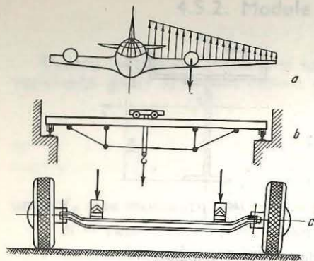
Fig. 5.1. Exemple de bare solicitate la încovoiere:
