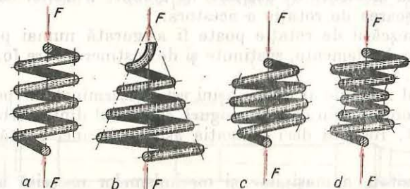
Fig. 10.8. Arcuri elicoidale:
