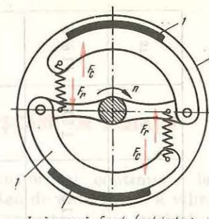
Fig. 12.10. Ambreiaj cu fricțiune centrifug.
