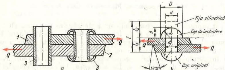
Fig. 8.3. Asamblare cu nituri: a — cu nituri tubulare: 1 și 2 — elementele îmbinării; 3 — nit tubular; b — cu nituri cilindrice.
