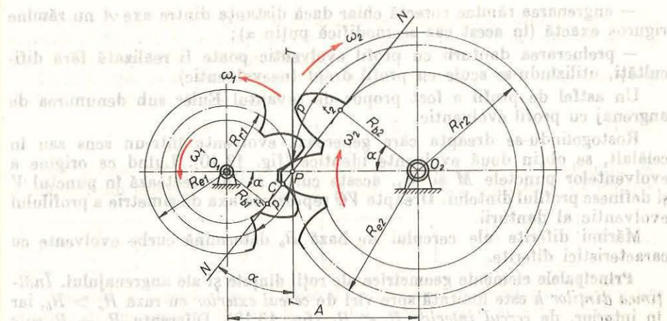
Fig. 13.11. Condiția de bază a angrenării cu raport de transmitere constant ( i = \text{constant} ).
