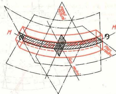
Fig. 5.18. Definirea diverselor elemente geometrice caracteristice unei bare solicitate la încovoiere.
