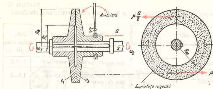
Fig. 12.7. Ambreiaj cu fricțiune având suprafețe plane.
