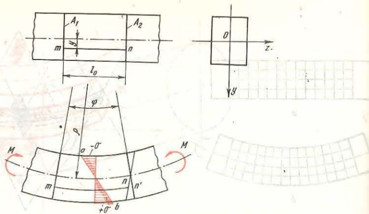
Fig. 5.19. Element de bară dreaptă supus la încovoiere.
