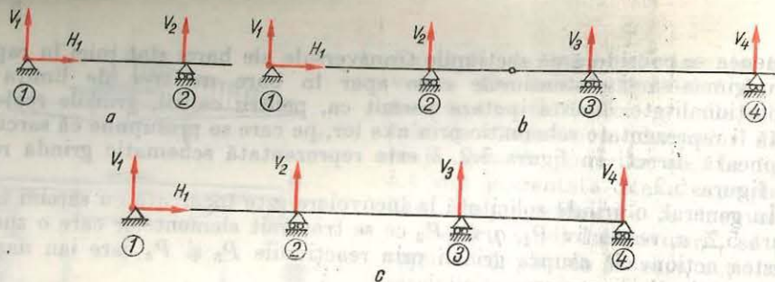
Fig. 5.5. Grinzi pe două sau mai multe reazeme: a — grindă pe două reazeme cu consolă; b — grindă cu patru reazeme articulată; c — grindă continuă pe patru reazeme.
