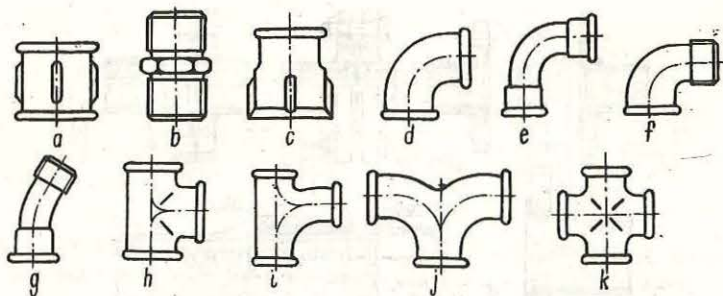
Fig. 14.5. Reprezentarea schematică a diferitelor forme uzuale de fittinguri.
