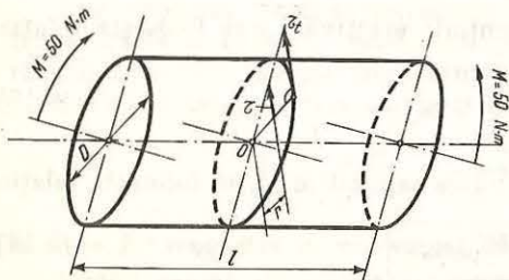
Fig. 6.6. Exemplu de calcul al unei bare drepte de secțiune circulară supusă la sollicitarea de răsucire.
