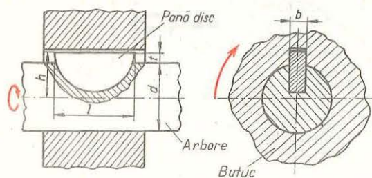
Fig. 9.5. Asamblarea cu pană-disc, STAS 1012-77.
