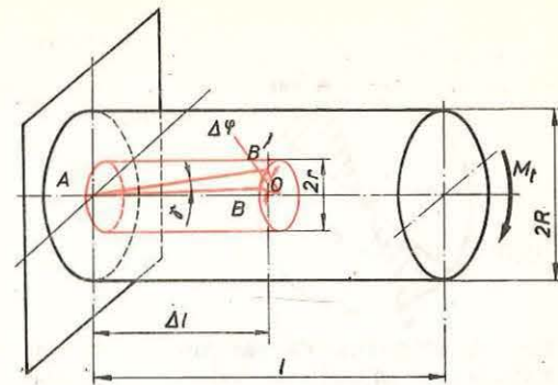
Fig. 6.3. Deformațiile mici ale barei de secțiune circulară, încăstrată la o extremitate și solicitată la răsucire prin acțiunea unui cuplu de moment M_t , aplicat în extremitatea liberă.
