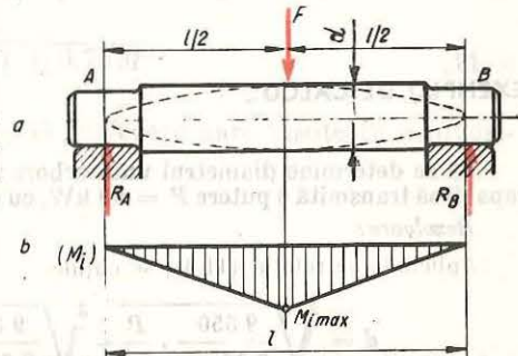
Fig. 11.6. Schema încărcării și diagrama de momente încovoiatoare M_i ale unei osii.
