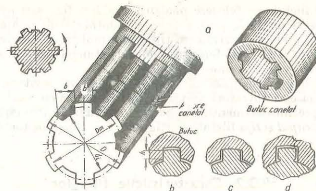
Fig. 9.6. Piese canelate:
