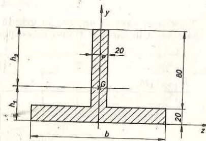
Fig. 5.21. Grindă de fontă cu secțiunea T.
