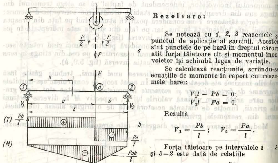
Fig. 5.10. Grindă simplu rezemată încărcată cu o sarcină concentrată:
