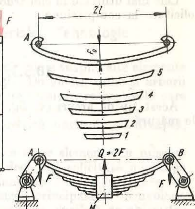
Fig. 10.7. Arc lamelar dublu cu foi multiple utilizat în construcția autovehiculelor:
