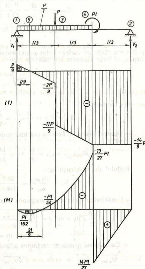
Fig. 5.20. Grindă simplu rezemată încărcată complex.
