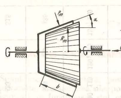
Fig. 12.9. Ambreiaj cu fricțiune conic.
