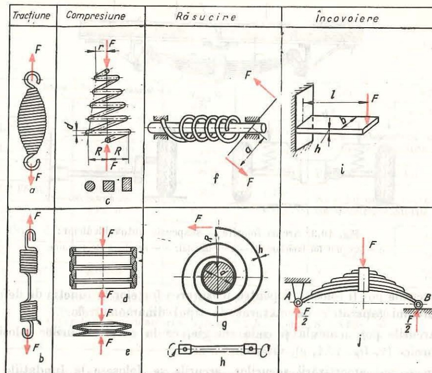
Fig. 10.1. Cele mai uzuale tipuri constructive de arcuri:
