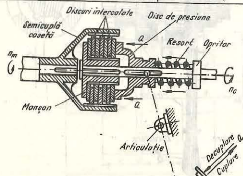
Fig. 12.8. Ambreiaj elastic cu discuri multiple.
