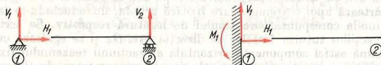
Fig. 5.3. Grindă dreaptă articulată la un capăt și rezemată liber de celălalt.
