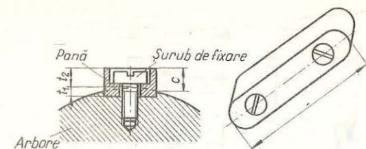
Fig. 9.4. Asamblarea cu pană longitudinală paralelă, STAS 1006-71.
