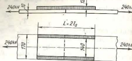
Fig. 3.10. Îmbinare sudată.
