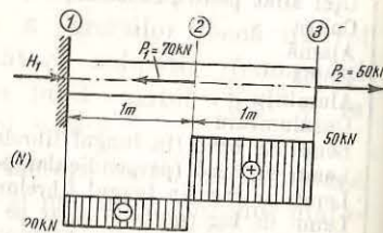
Fig. 2.2. Grindă solicitată de mai multe sarcini axiale.
