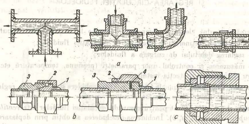
Fig. 14.4. Secțiuni prin diverse fittinguri și racorduri: a — fittinguri; b — îmbinări cu racorduri olandeze (1 — șut; 2 — piuliță cu filet interior; 3 — piuliță cu filet exterior; 4 — garnitură); c — piuliță olandeză cu inel conic.
