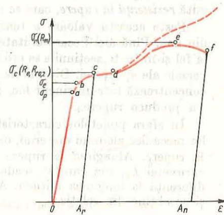
Fig. 1.8. Curba caracteristică a oțelului moale.
