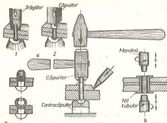
Fig. 8.1. Principalele faze tehnologice ale nituirii: a — nituire manuală; 1 — stringerea pieselor; 2 — refularea tijei și formarea capului de închidere; b — nituire mecanică prin mandrinare; c — nituire cu exploziv.
