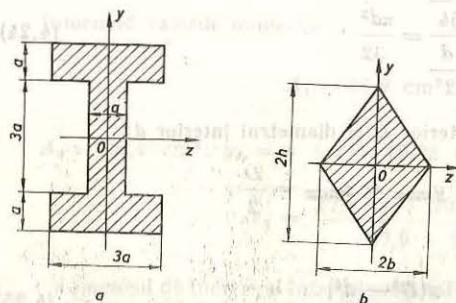
Fig. 4.10. Suprafețe compuse.
