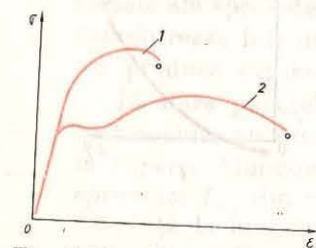
Fig. 1.11. Comportarea oțelului moale la sarcini aplicate static (1) și la variația rapidă a acestora (2).
