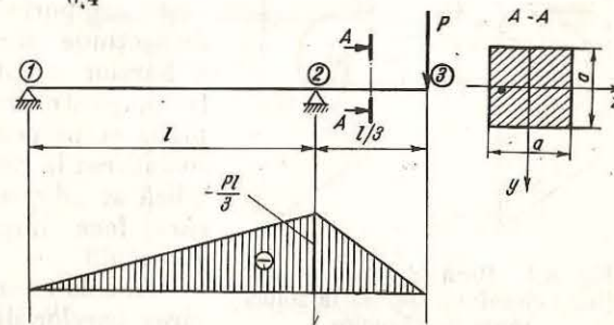
Fig. 5.23. Grindă dreaptă în consolă simplu rezemată, cu o sarcină concentrată pe capătul liber.
