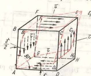
Fig. 1.6. Deformarea unui corp prin lunecare.
