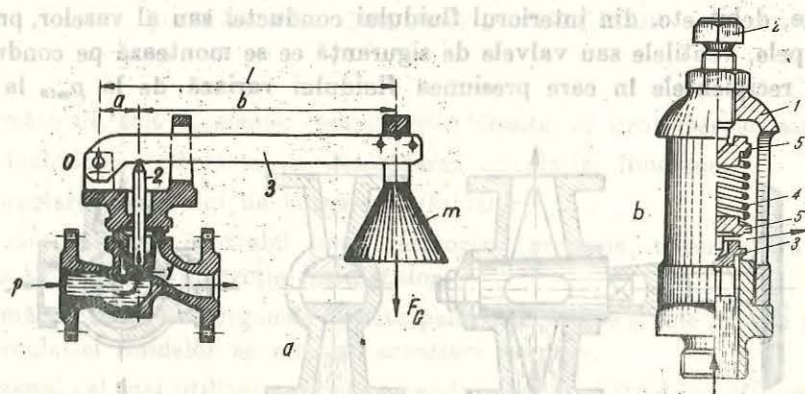
Fig. 14.9. Supape de siguranță pentru prevenirea creșterii presiunii: a - supapă cu pirghie și contragreutate; 1 - ventil; 2 - tijă; 3 - pirghie; b - supapă cu arc elicoidal; 1 - corpul supapei; 2 - șuruburi de reglare; 3 - ventil; 4 - arc; 5 - suporturile arcului.
