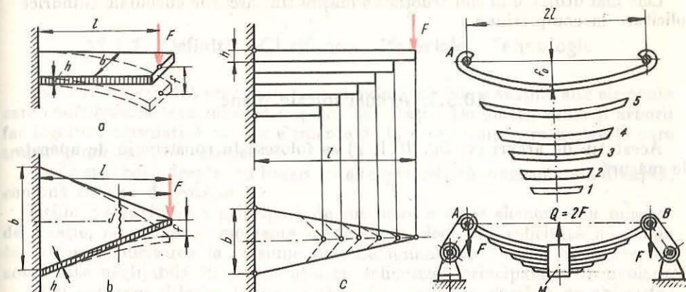
Fig. 10.6. Arcuri lamelare:
