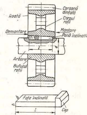
Fig. 9.3. Asamblarea cu pană longitudinală.
