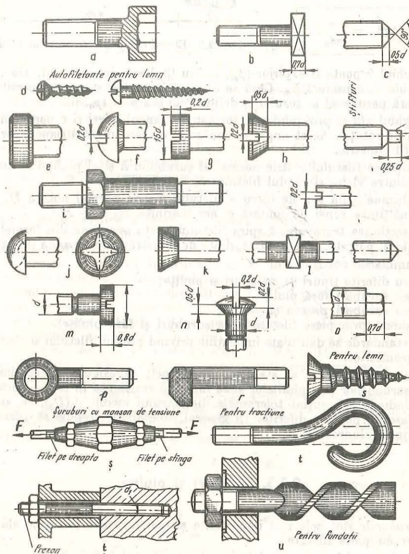
Fig. 9.10. Diferite forme constructive de șuruburi:
