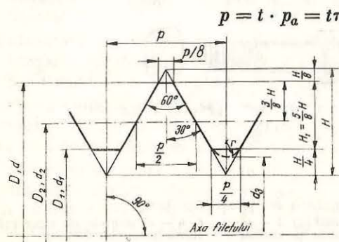
Fig. 9.8. Elementele geometrice de bază ale filetelui metric — după STAS 6371-73.
