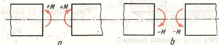
Fig. 5.9. Convenția de semne pentru momentul încovoietor: a — pozitiv; b — negativ.
