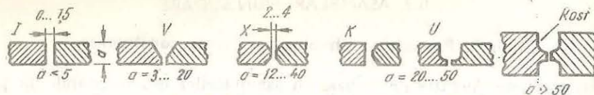
Fig. 8.8. Forma rostului cordonului de sudură.
