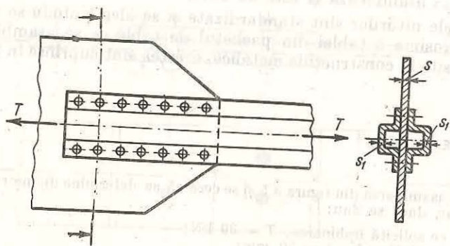
Fig. 3.6. Asamblarea nituită a unor piese din duraluminu.
