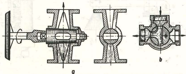
Fig. 14.7. Robinet cu cep sau cană:
