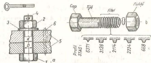
Fig. 9.7. Elementele asamblării cu piese filetate:
