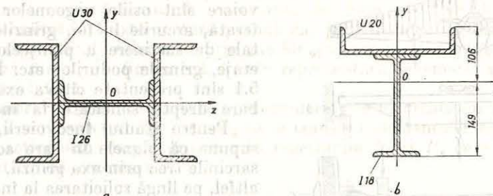
Fig. 4.11. Secțiuni compuse din profiluri laminate.
