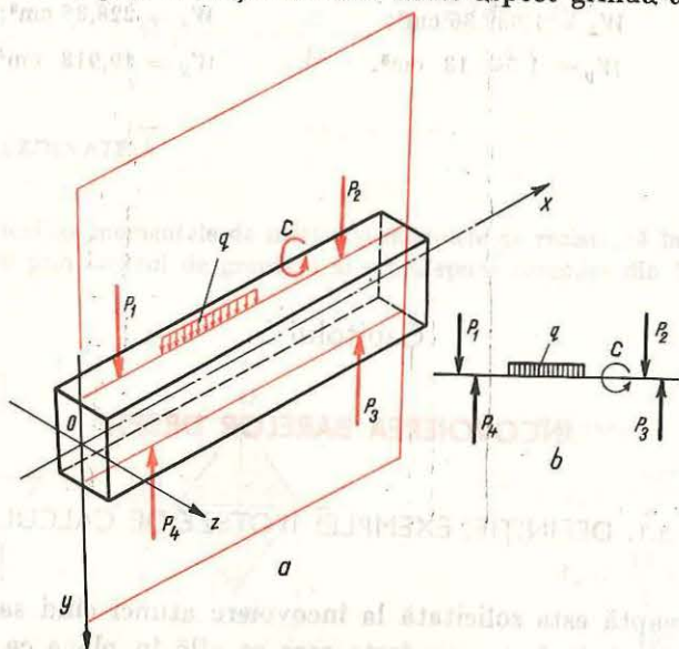
Fig. 5.2. Grindă solicitată la încovoiere cu sarcinile cuprinse în planul de simetrie.
