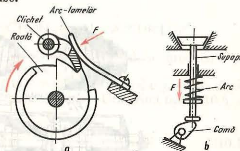
Fig. 10.2. Arcuri pentru crearea unei forțe de presiune constantă:
