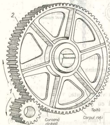
Fig. 13.8. Angrenaj cu roți dințate cilindrice cu dinți drepti: 1 — roată conducătoare; 2 — roată condusă.
