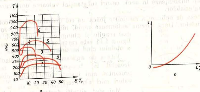
Fig. 1.9. Formă curbei caracteristice pentru câteva materiale:
