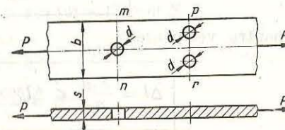
Fig. 2.3. Piesă cu o secțiune brută, două secțiuni nete ( m-n , p-r ) și o secțiune periculoasă ( p-r ).
