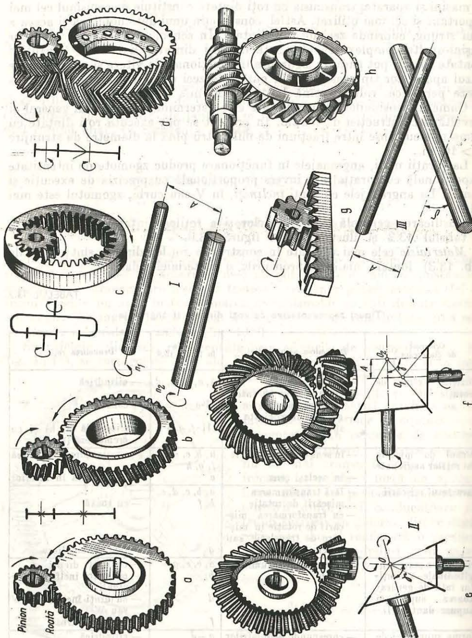
Fig. 13.9. Principalele tipuri de angrenaje cu roți dințate.
