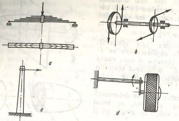
Fig. 1.2. Exemple de piese supuse la sollicitări simple: a, c - la încovoiere; b, d - la răsucire.
