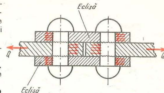
Fig. 8.4. Asamblare nituită cap la cap cu două eclise.
