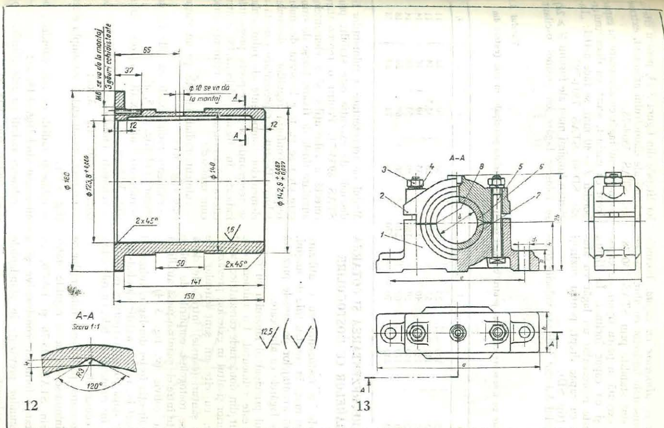
Fig. 3.12. Bucșă cu guler prevăzută cu gaură și canal de ungere.
