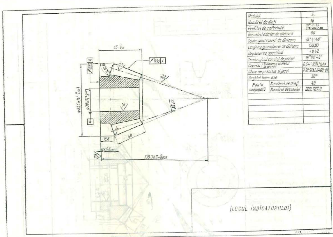
Fig. 3.36. Indicarea elementelor danturii pe desen la roțile dințate conice. Completarea tabelului cu elementele caracteristice.
