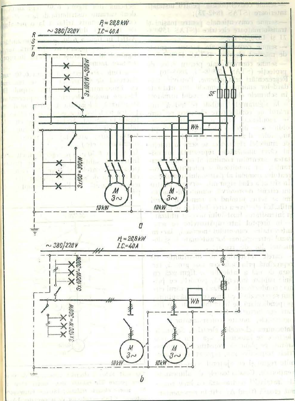
Fig. 6.30. Reprezentarea unei instalații electrice a — schemă electrică trifilară; b — în schemă monofilară de forță și iluminat:
