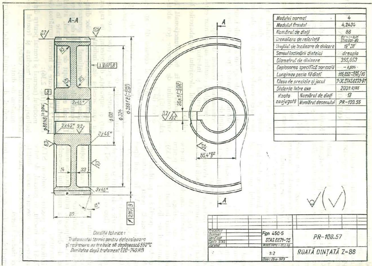
Fig. 3.35. Desenul definitiv (de execuție) al unei roți dințate cilindrice cu dinți înclinați.
