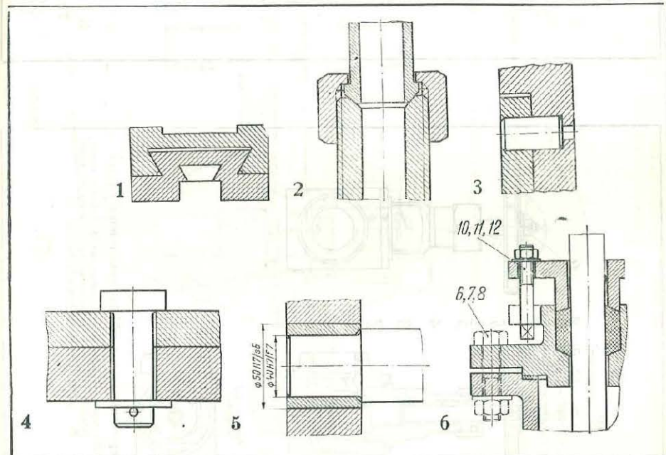
Fig. 4.1. Hașurarea a două piese asamblate.
