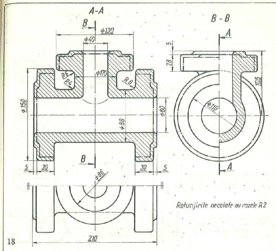
Fig. 6.18. Desenul de semifabricat al teului cu flanșă din figura 6.16.
