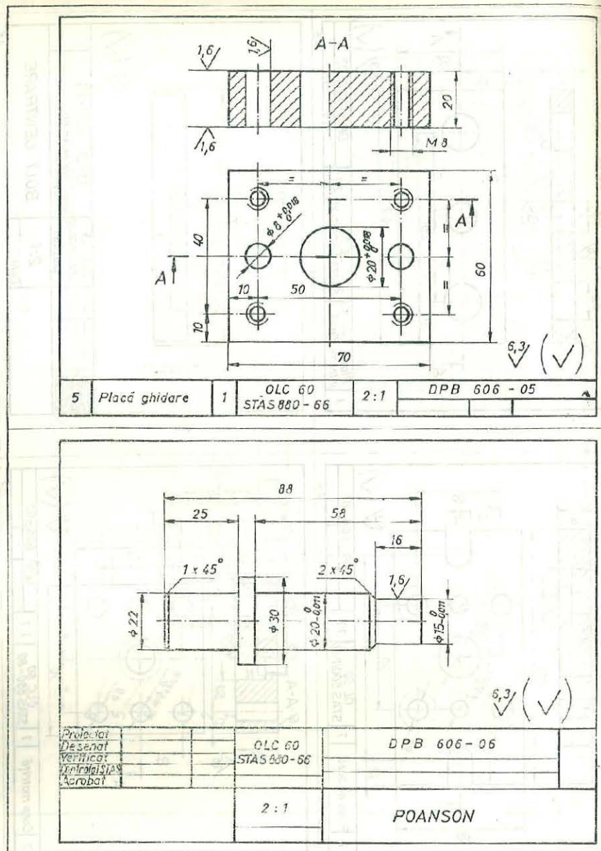
Fig. 4.22. Piese componente ale dispozitivului din figura 4.20. (Desene la scară pe formate A5.)
