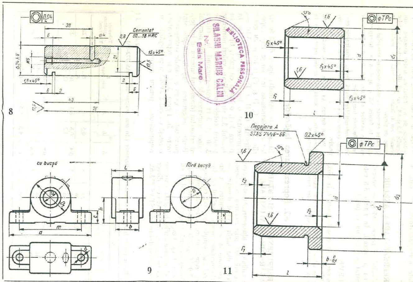
Fig. 3.8. Reprezentarea și cotarea unui ax.
