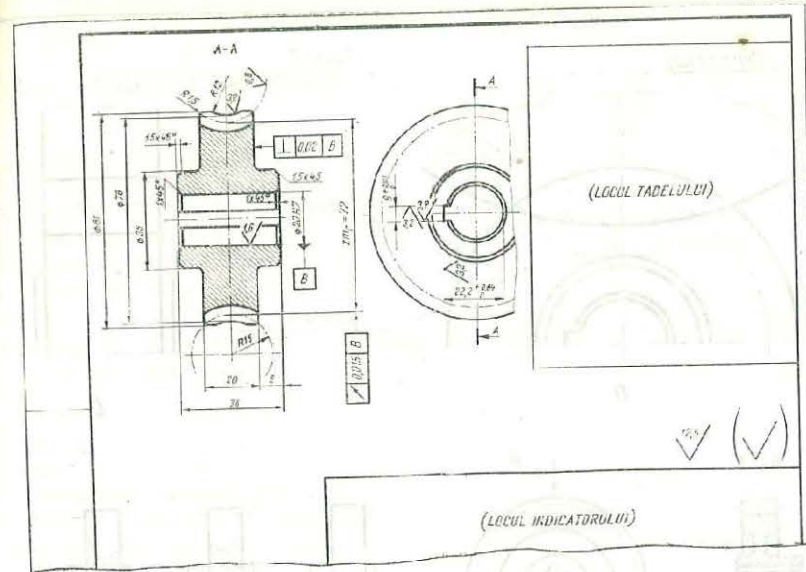
Fig. 3.40. Desenul de execuție al roții melcate.
