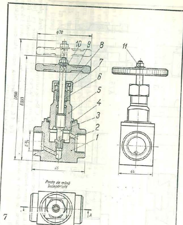
Fig. 4.7. Reprezentarea ansamblului unui robinet cu ac:
