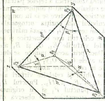
Fig. 7.1. Triunghiul urmelor planului în reprezentarea izometrică.
