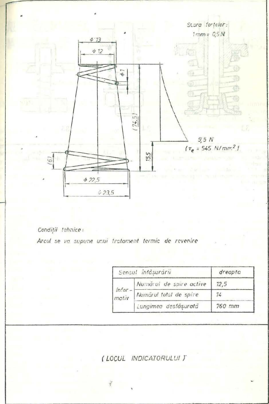
32. Arc elicoidal conic de compresiune.
