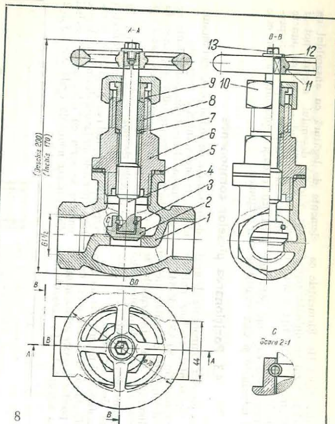
Fig. 4.8. Reprezentarea ansamblului unui robinet cu ventil:
