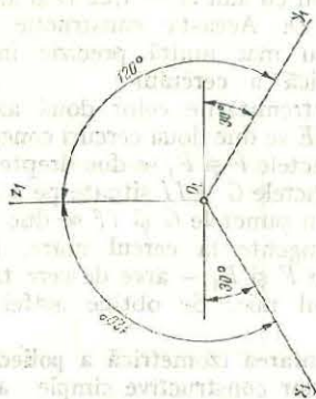
Fig. 7.3. Unghiurile din axe în reprezentarea izometrică.
