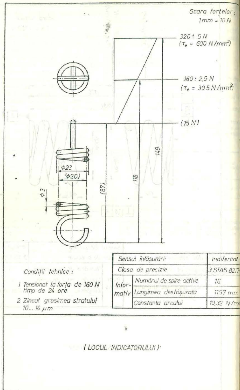
Fig. 2.31. Arc elicoidal cilindric, de tracțiune, pretensionat.
