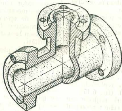
Fig. 6.16. Desenul de execuție al unui teu cu flanșe cilindrice.
