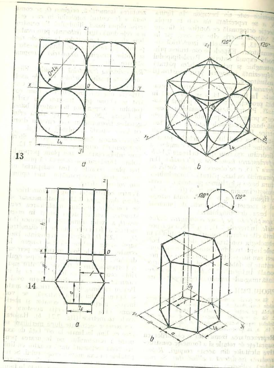
Fig. 7.13. Proiecția ortogonală a unui cub cu cercuri înscrise pe cele trei fețe văzute și reprezentarea izometrică.
