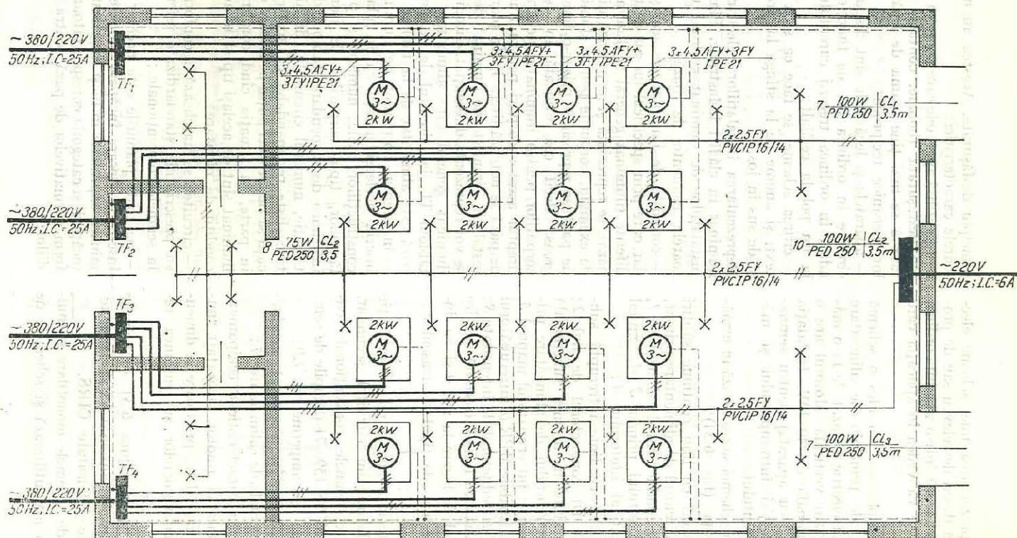
Fig. 6.32. Planul instalației de forță și iluminat într-un atelier de presă mecanică (schemă monofilară)
