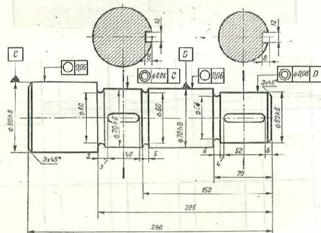
Fig. 1.16. Înscrisura cotei, urmată de simbolurile celor două cimpuri de toleranță.
