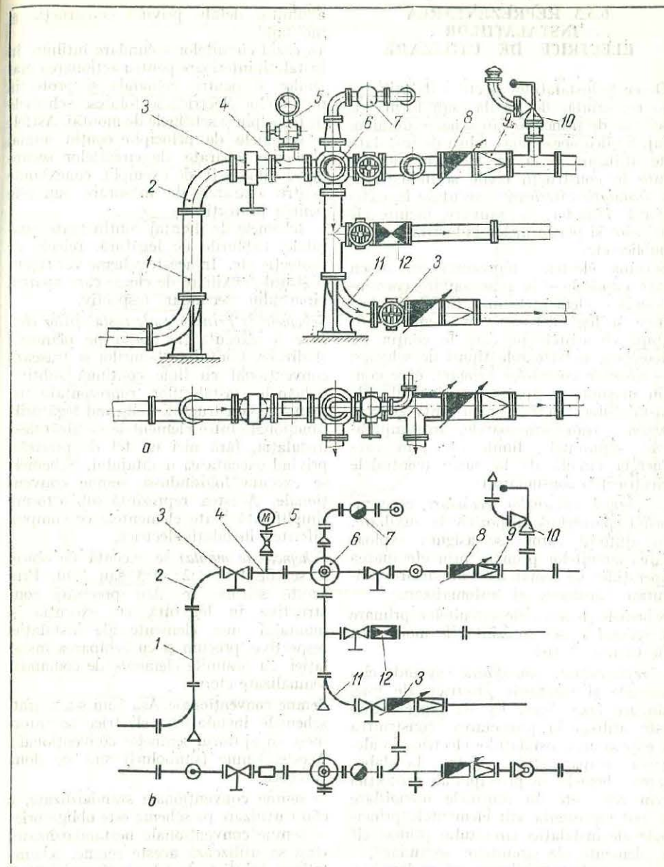
Fig. 6.29. Instalație pentru transportul aburului sub presiune: 1 - tub cu flanșe; 2 - cot cu flanșe; 3 - robinet cu sarter; 4 - ramificații cu flanșe; 5 - manometru; 6 - ramificație
