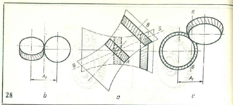
Fig. 3.28. Angrenaj hiperboloidal (hipoid).
