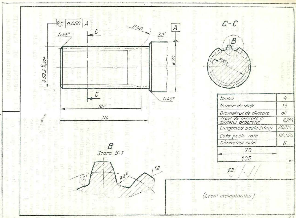
Fig. 2.25. Desenul de execuție al unui capăt de arbore prevăzut cu caneluri în evolută.
