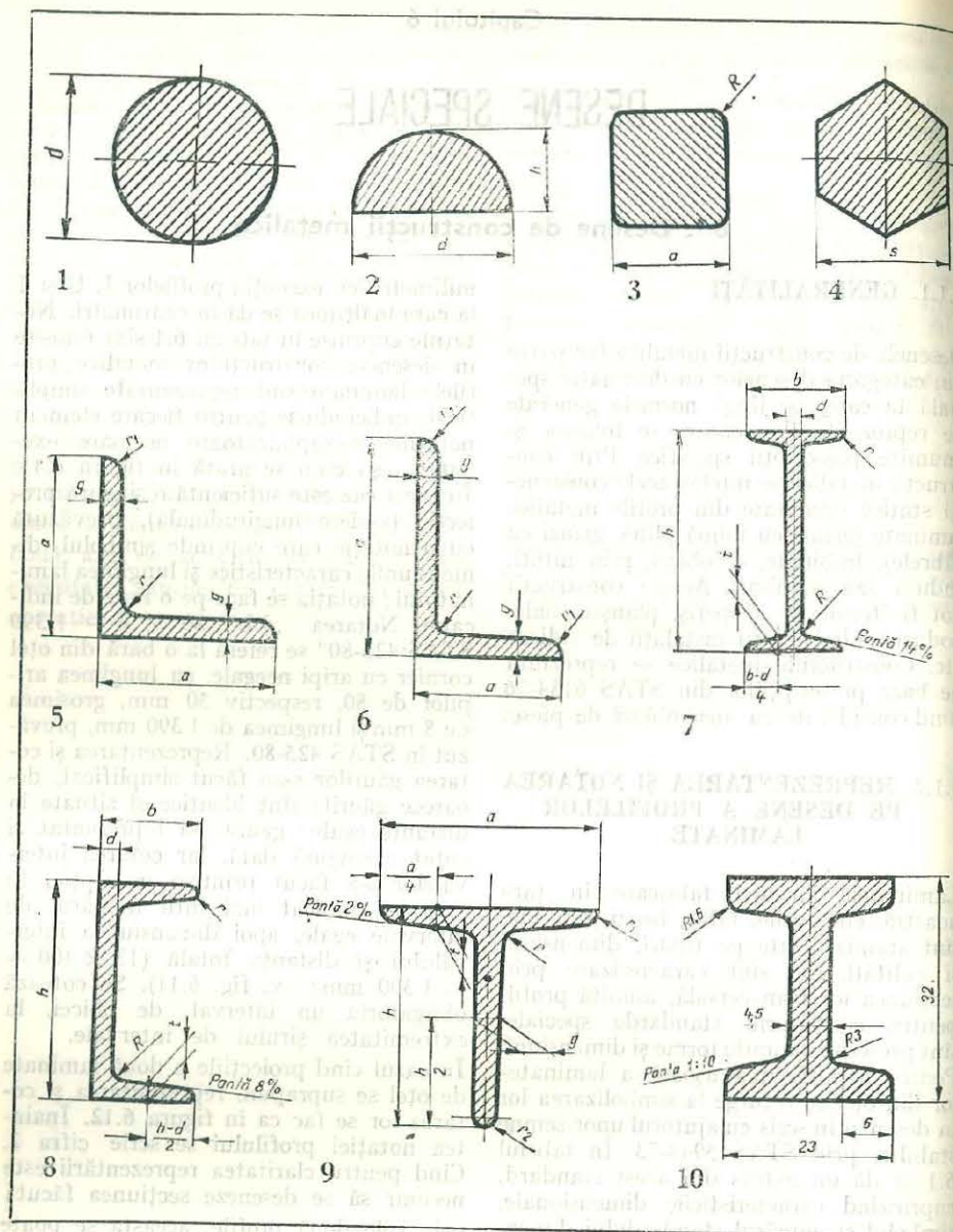
Fig. 6.1. Profil laminat rotund. Fig. 6.2. Profil laminat semirotund. Fig. 6.3. Profil laminat pătrat. Fig. 6.4. Profil laminat hexagonal. Fig. 6.5. Cornier cu aripi egale.
