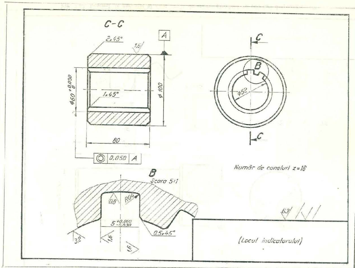
Fig. 2.24. Desenul de execuție al unui butuc prevăzut cu caneluri dreptunghiulare.
