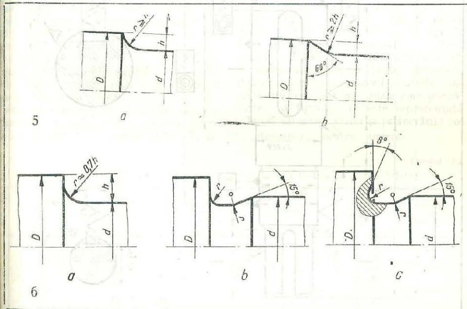
Fig. 3.5. Racordarea arborilor în trepte, fără unăr de sprijin:
