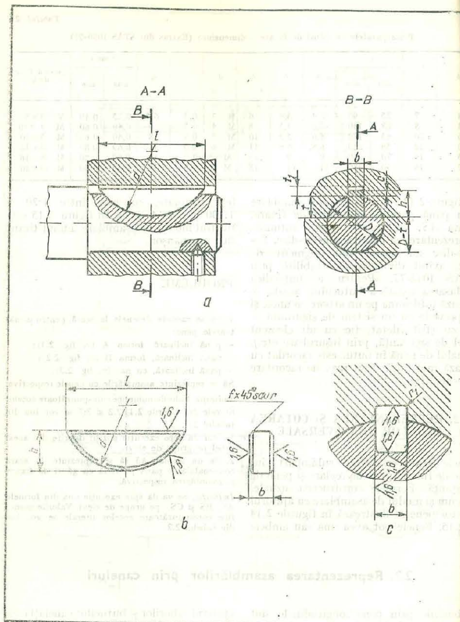
Fig. 2.13. Pană-disc:
