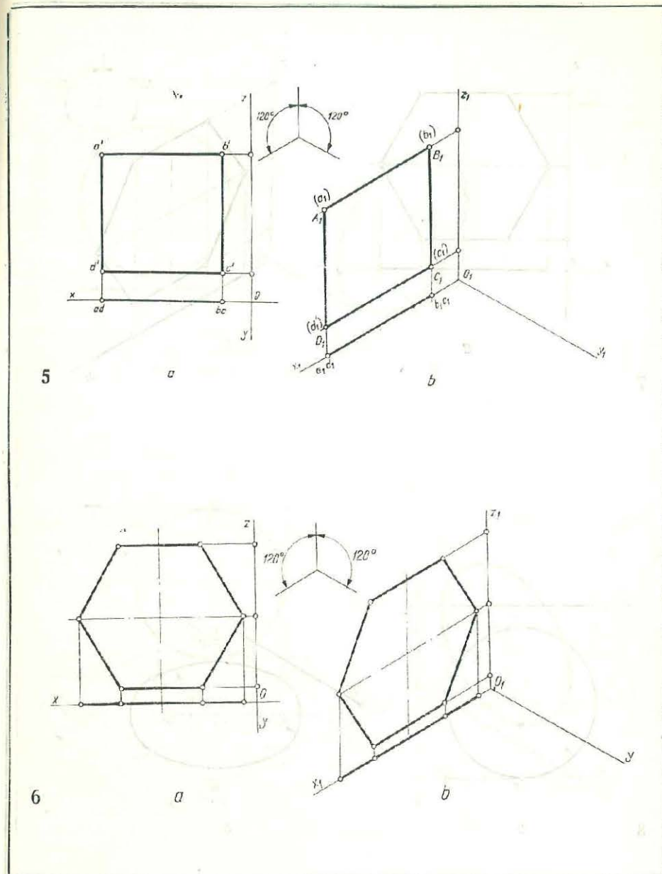
Fig. 7.5. Dubla proiecție ortogonală a unui pătrat conținut în planul vertical de proiecție și reprezentarea izometrică.
