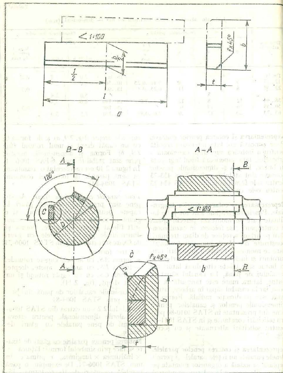
Fig. 2.7. Pană tangentă:
