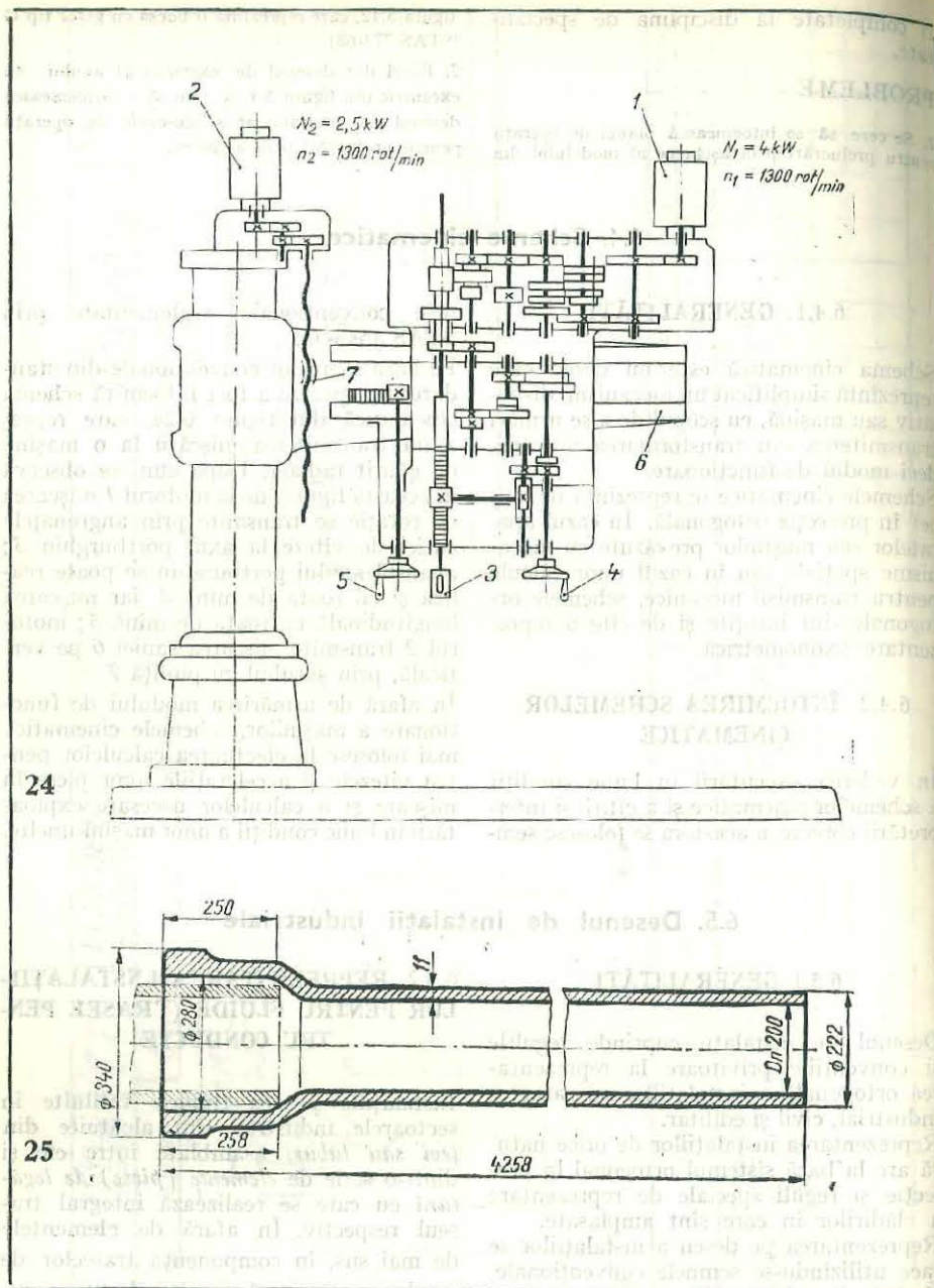
Fig. 6.24. Schema cinematică a unei mașini de găurit radiale.
