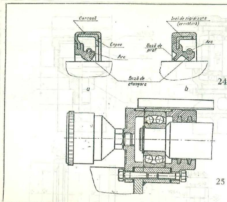
Fig. 3.24. Inel de etanșare din cauciuc: a - cu carcasă și arc; b - cu inel de rigidizare, arc și buză de praf.
