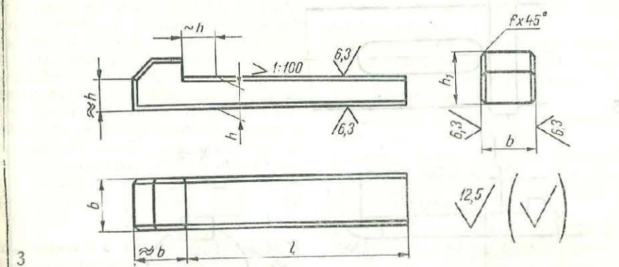
Fig. 2.1. Pană înclinată fără nas, forma A, cu capete rotunde.
