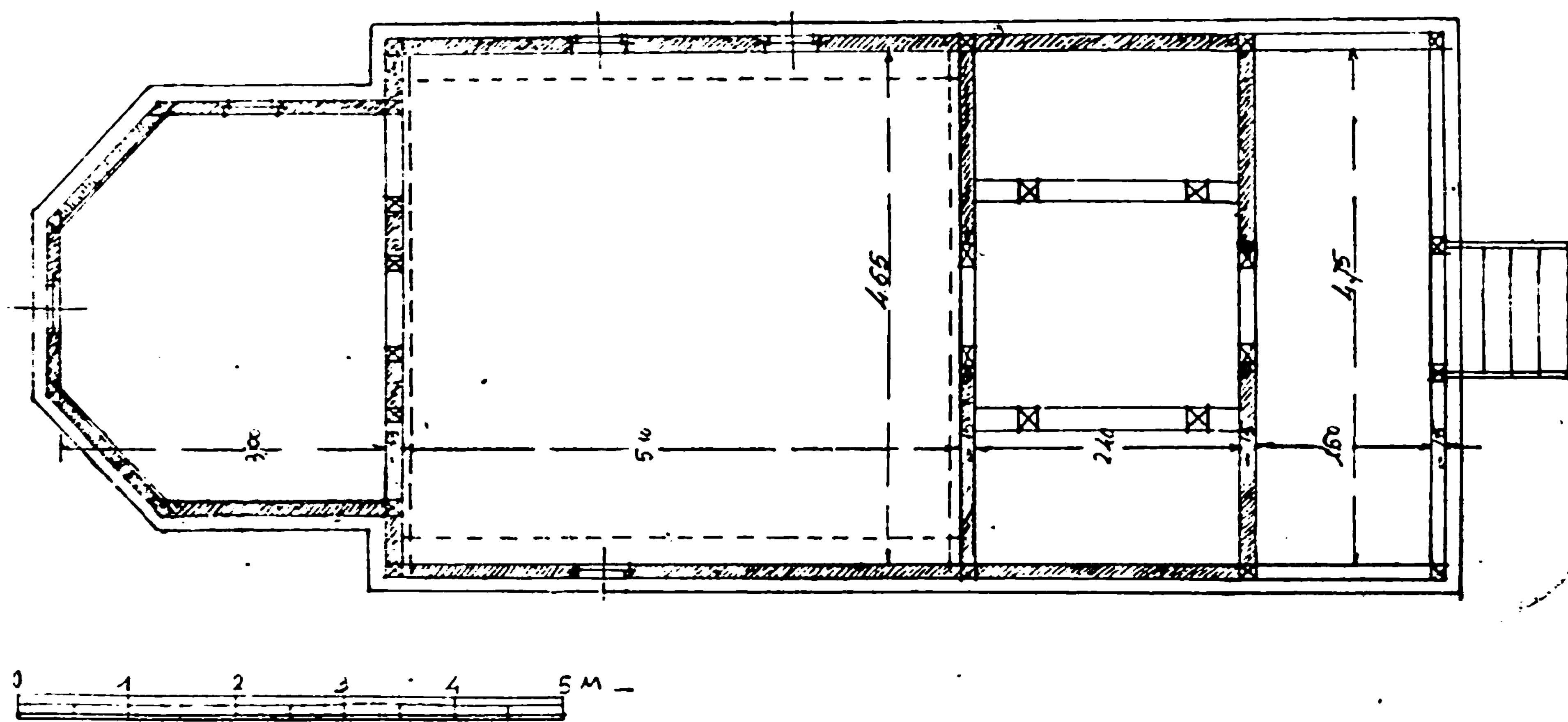
Planul bisericii de lemn din Mihăești-Capul Dealului (Vâlcea).
