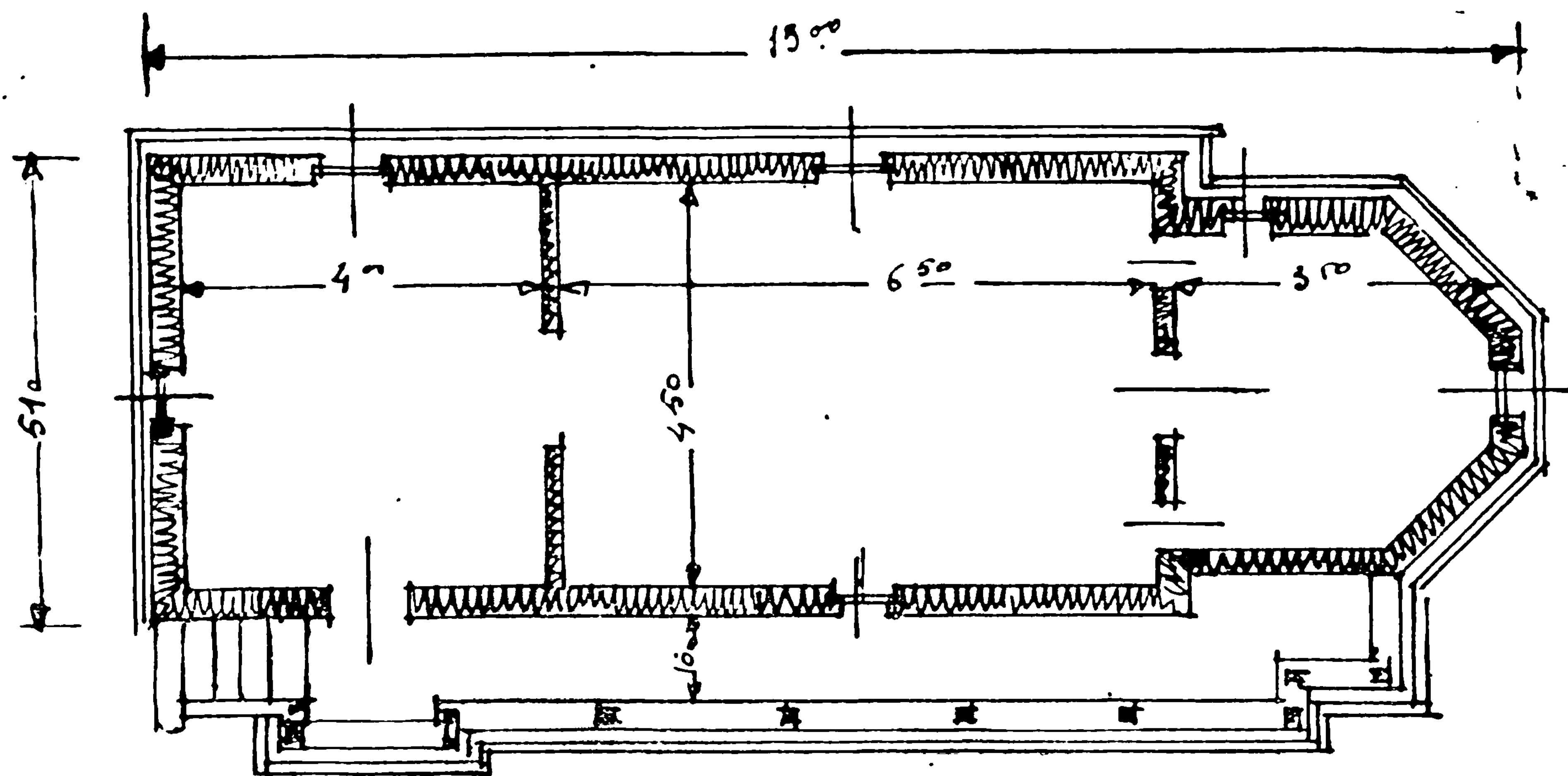
SCHITUL DRAGOSLAVELE. -- Planul Bisericii.
